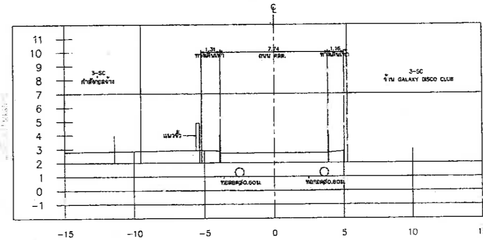
รูปตัดที่ 12 0+275
