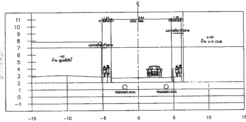
รูปตัดที่ 11 0+250
