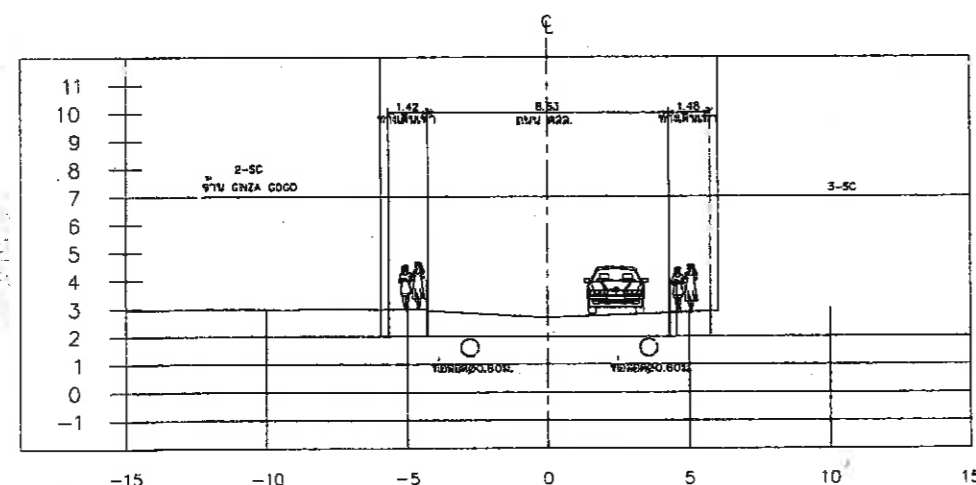
รูปตัดที่ 9 0+200
