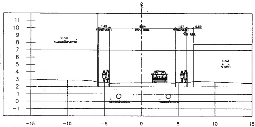
รูปตัดที่ 2 0+025
