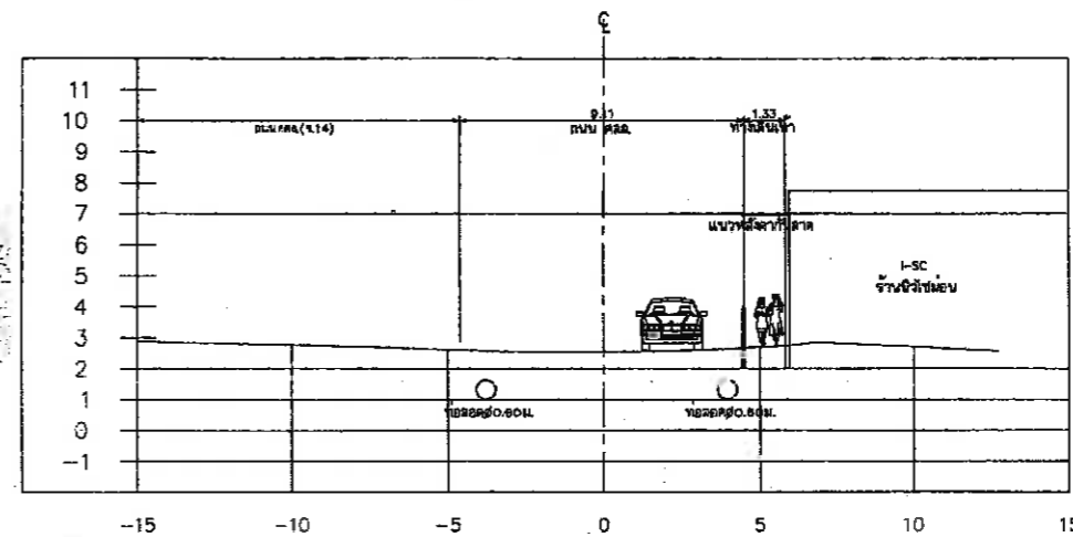
รูปตัดที่ 5 0+100
