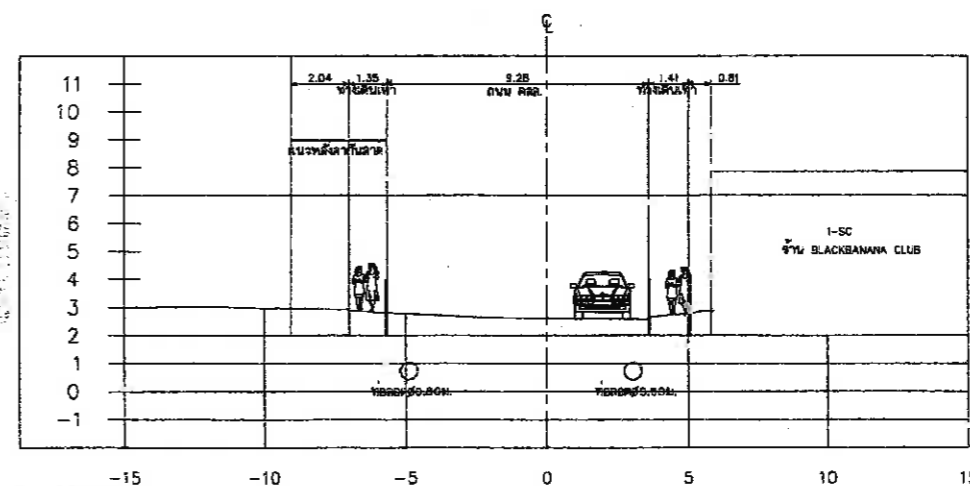
รูปตัดที่ 6 0+125
