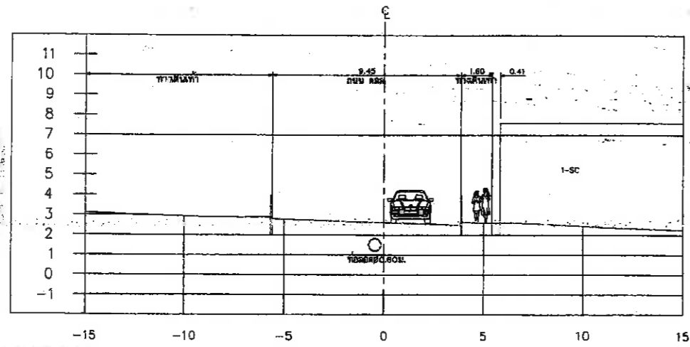
รูปตัดที่ 1 0+000
