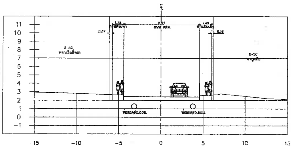
รูปตัดที่ 3 0+050
