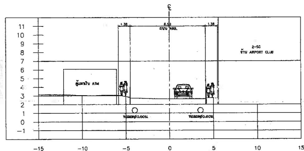
รูปตัดที่ 8 0+175
