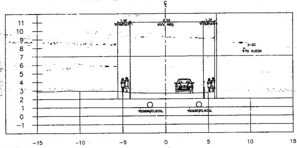
รูปตัดที่ 10 0+225
