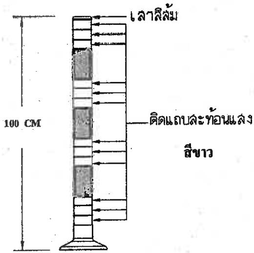
เสาเข็มลูก (สี่เหลี่ยม)
