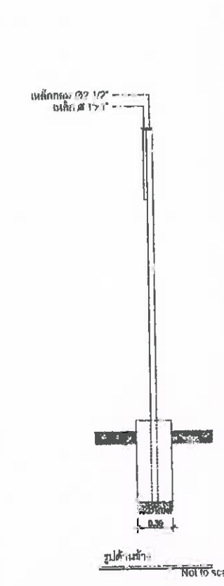
แบบแปลนค้ำยันแสดงรายละเอียดเกี่ยวกับงานก่อสร้าง กรณีอยู่ในระหว่างดำเนินการก่อสร้าง
