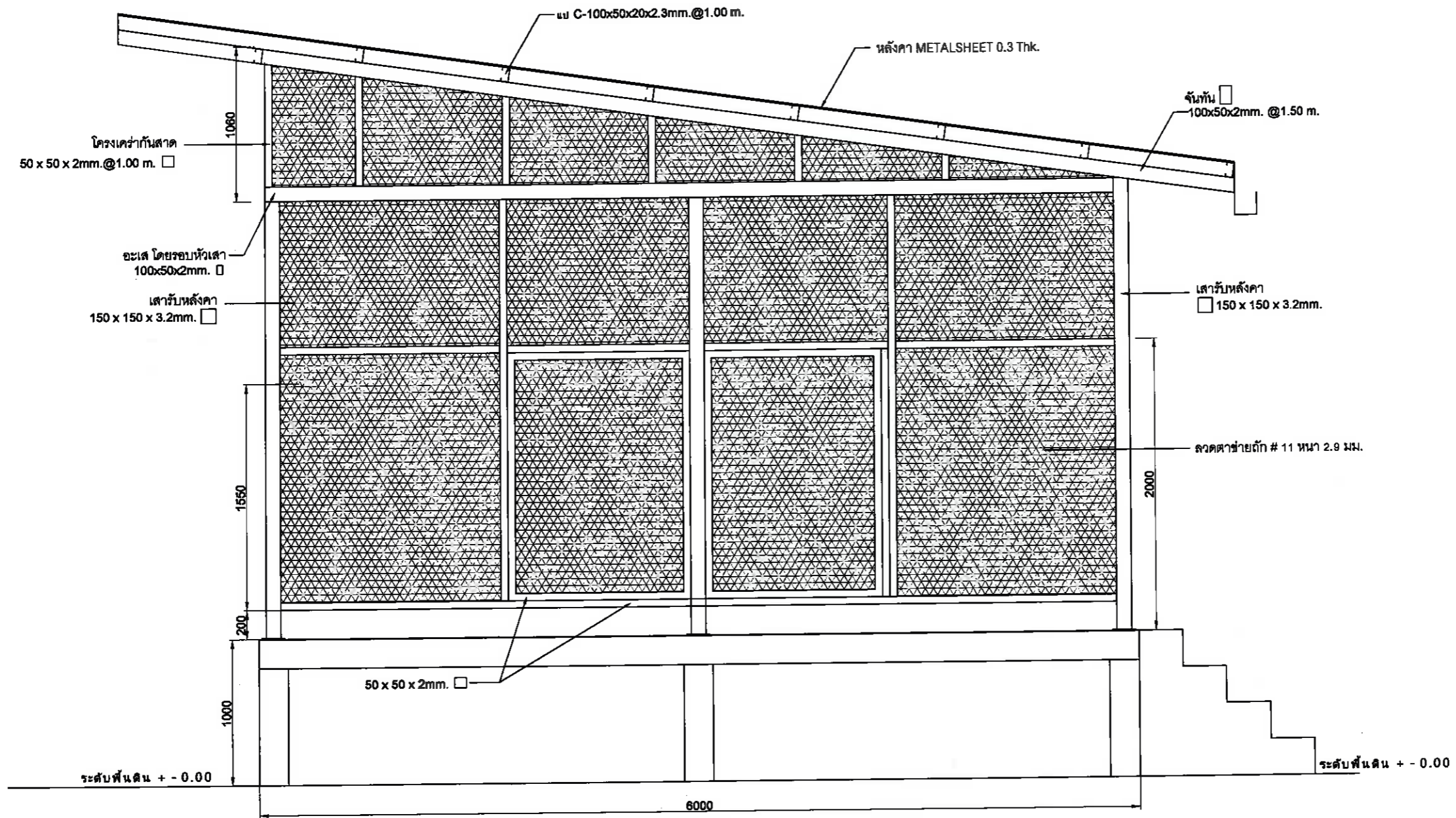
รูปด้าน D - D
