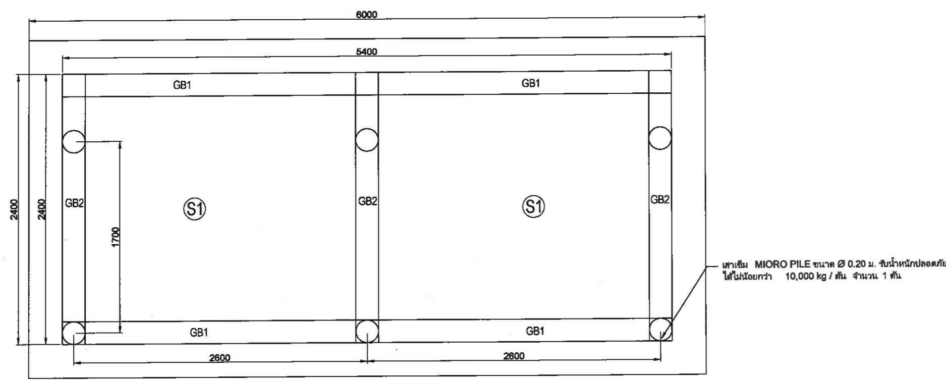
แปลนฐานราก SCALE 1:100
