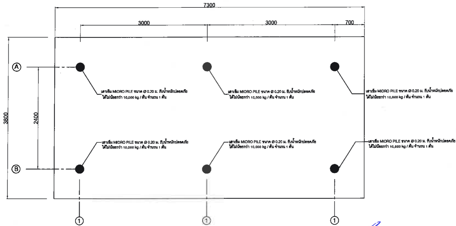
แปลนเสาเข็ม SCALE 1:100
