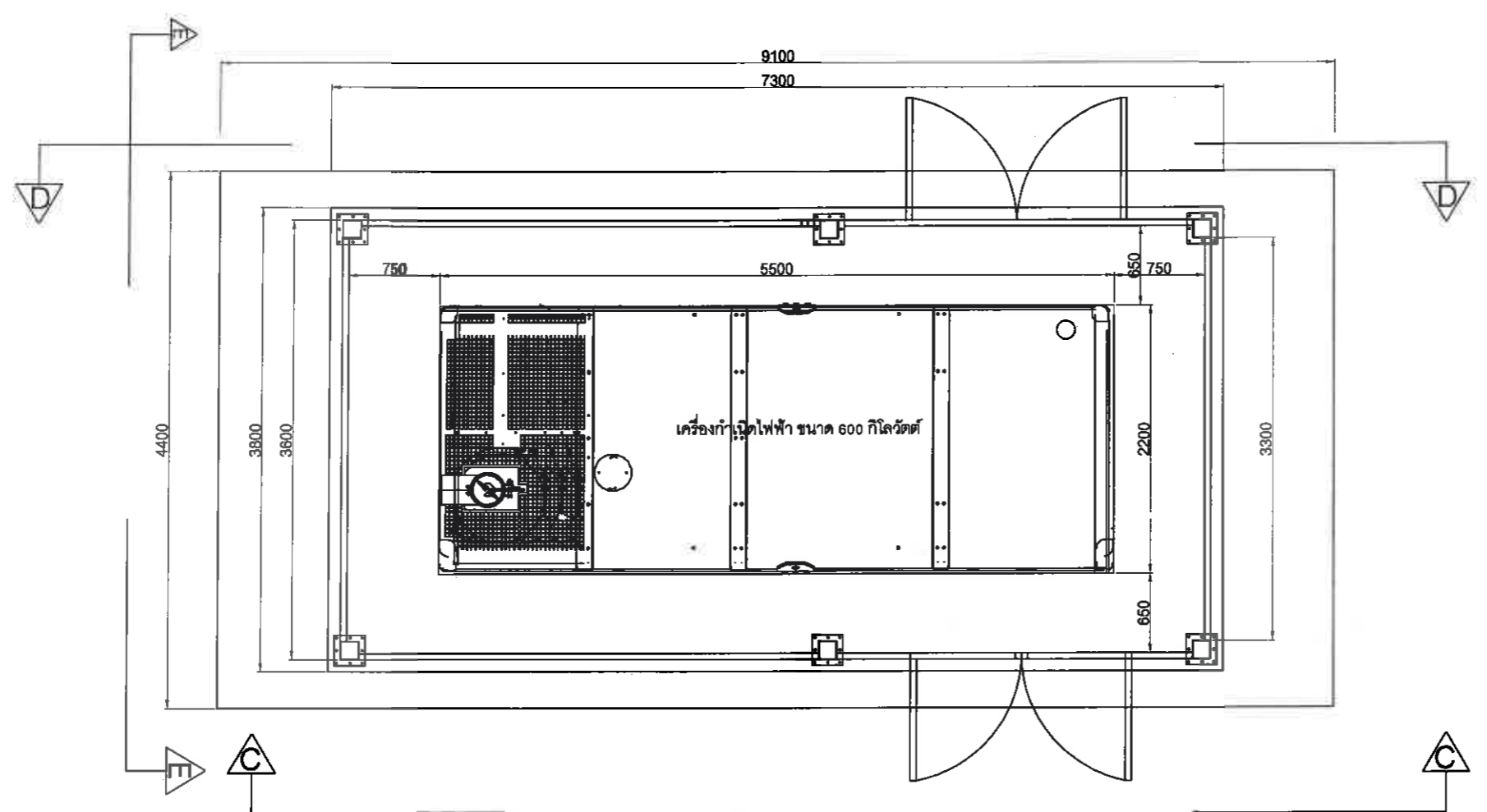
แปลนโรงควบคุมเครื่องกำเนิดไฟฟ้า SCALE 1:100
