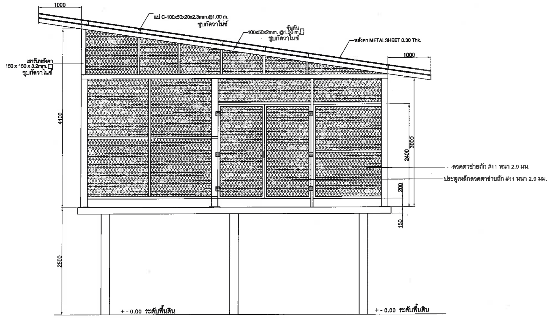
รูปด้าน D-D SCALE 1:100
