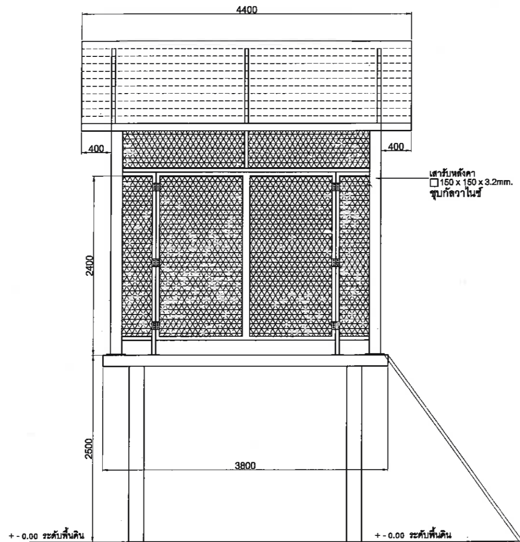
รูปด้าน E-E SCALE 1:100
