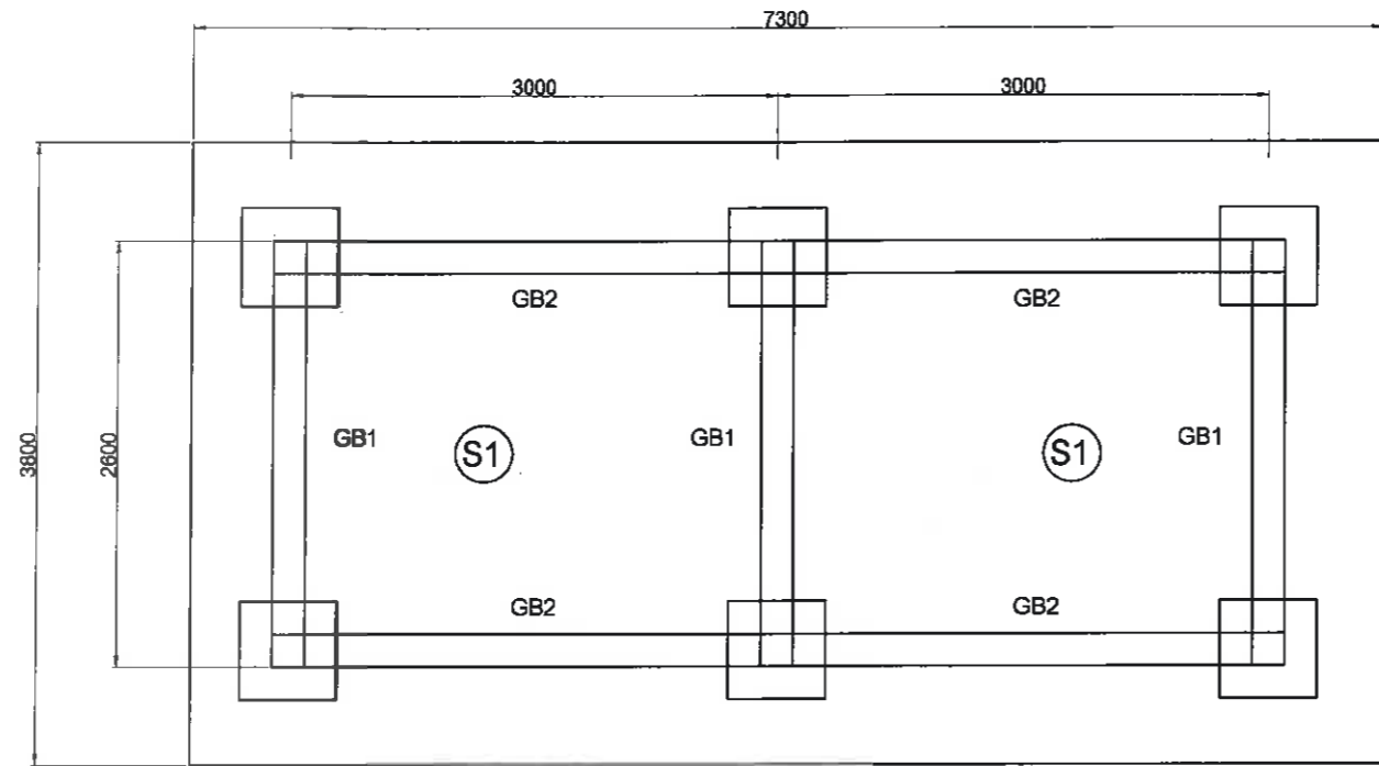
แปลน คาน SCALE 1:100
