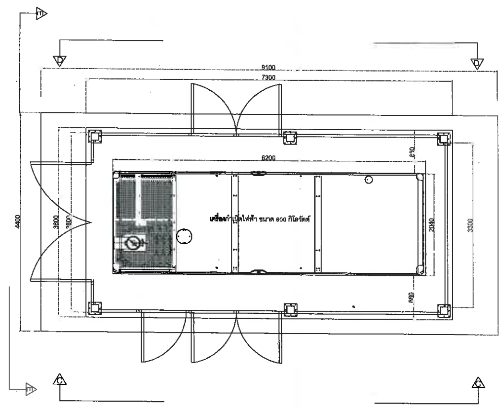
แปลนโรงควบคุมเครื่องกำเนิดไฟฟ้า SCALE 1:100
