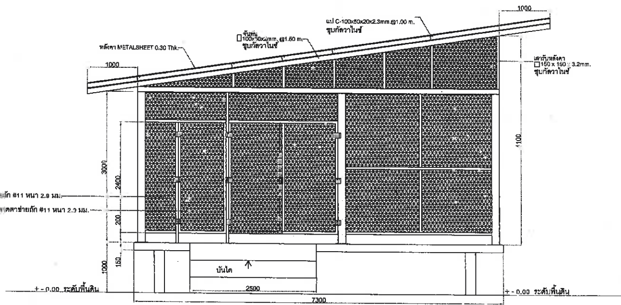
รูปด้าน C-C SCALE 1:100
