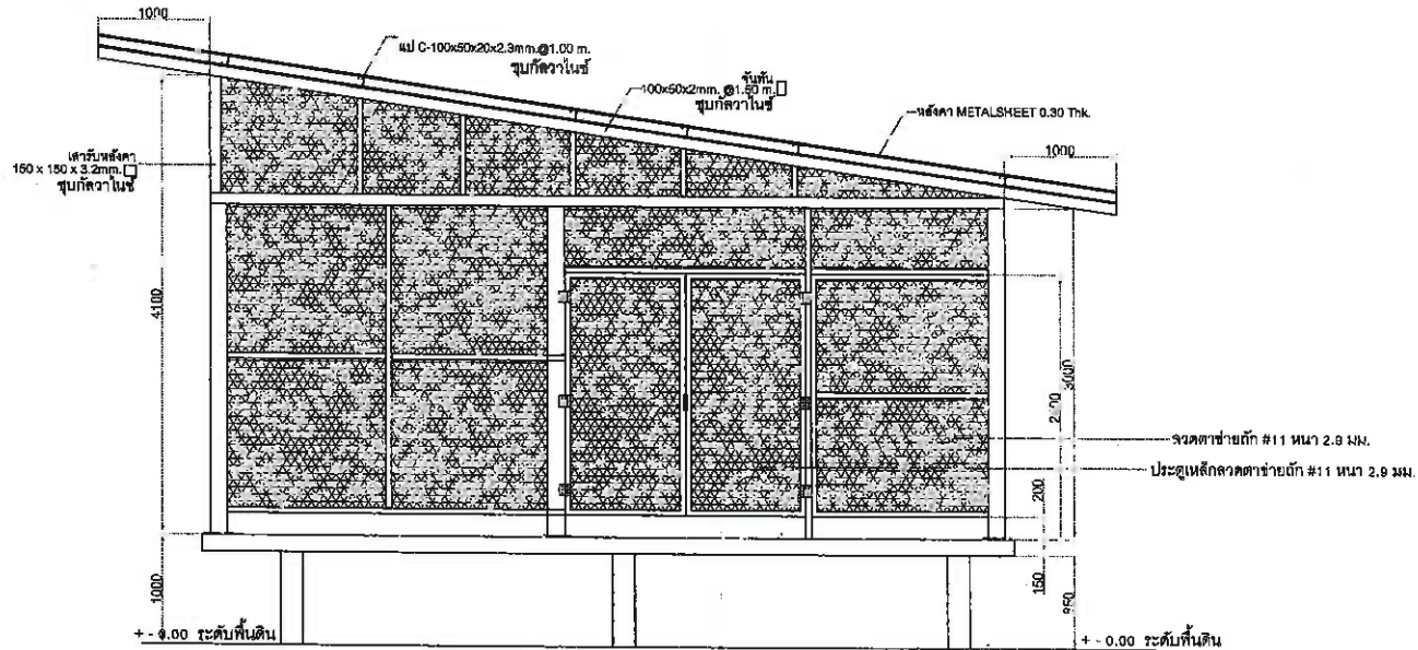
รูปด้าน D - D SCALE 1/100
