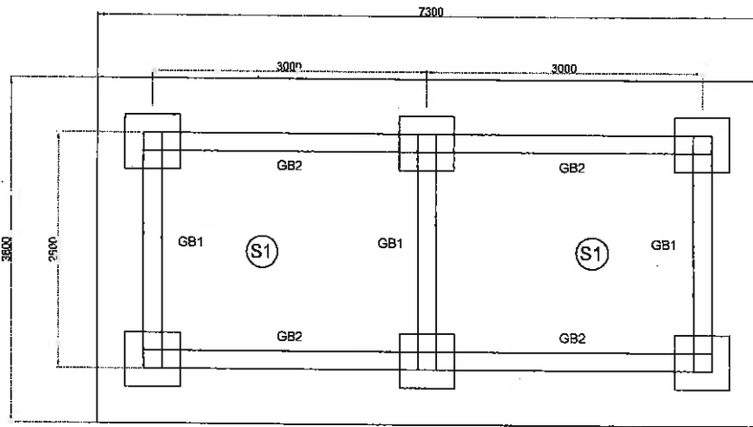
แปลน คาน SCALE 1:100
