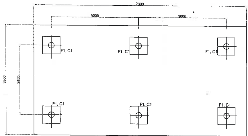
แปลนฐานราก SCALE 1:100
