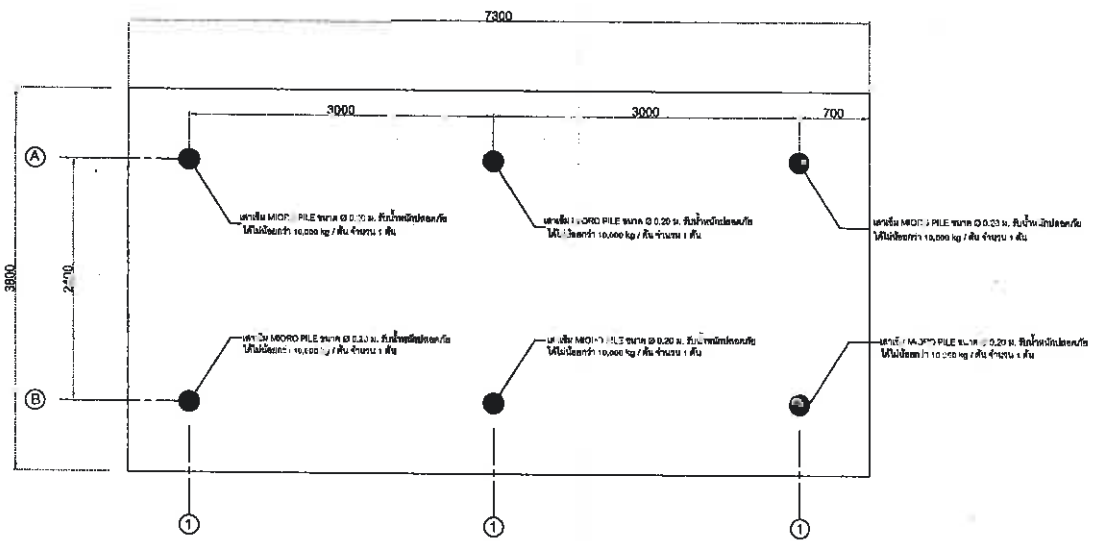
แปลนเสาเข็ม SCALE 1:100
