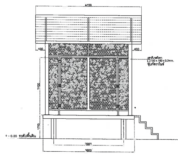
รูปด้าน C - C SCALE 1:100
