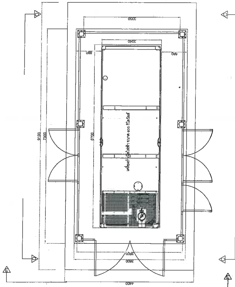
แปลนโครงสร้างเครื่องกำเนิดไฟฟ้า SCALE 1:100
