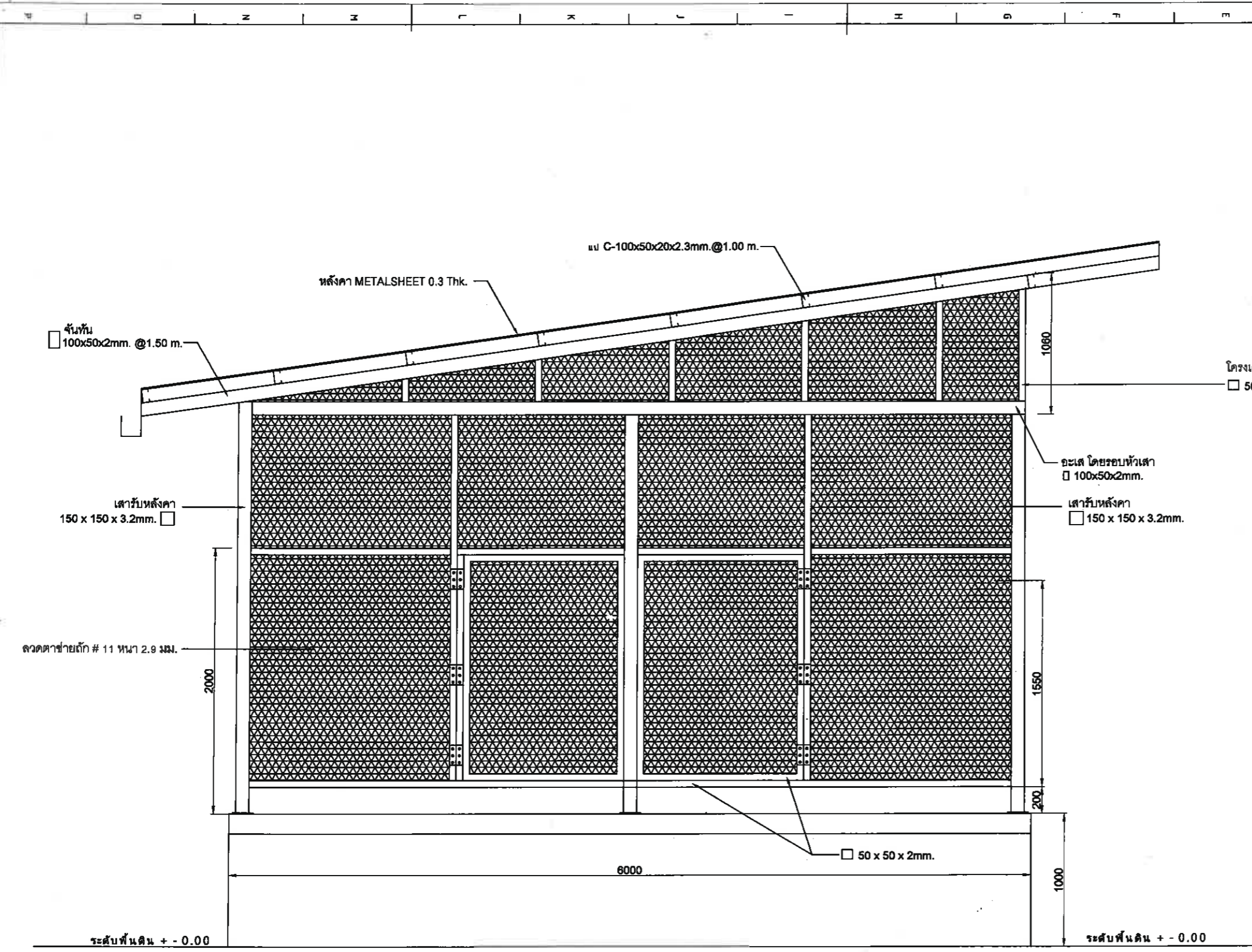
รูปด้าน C - C
