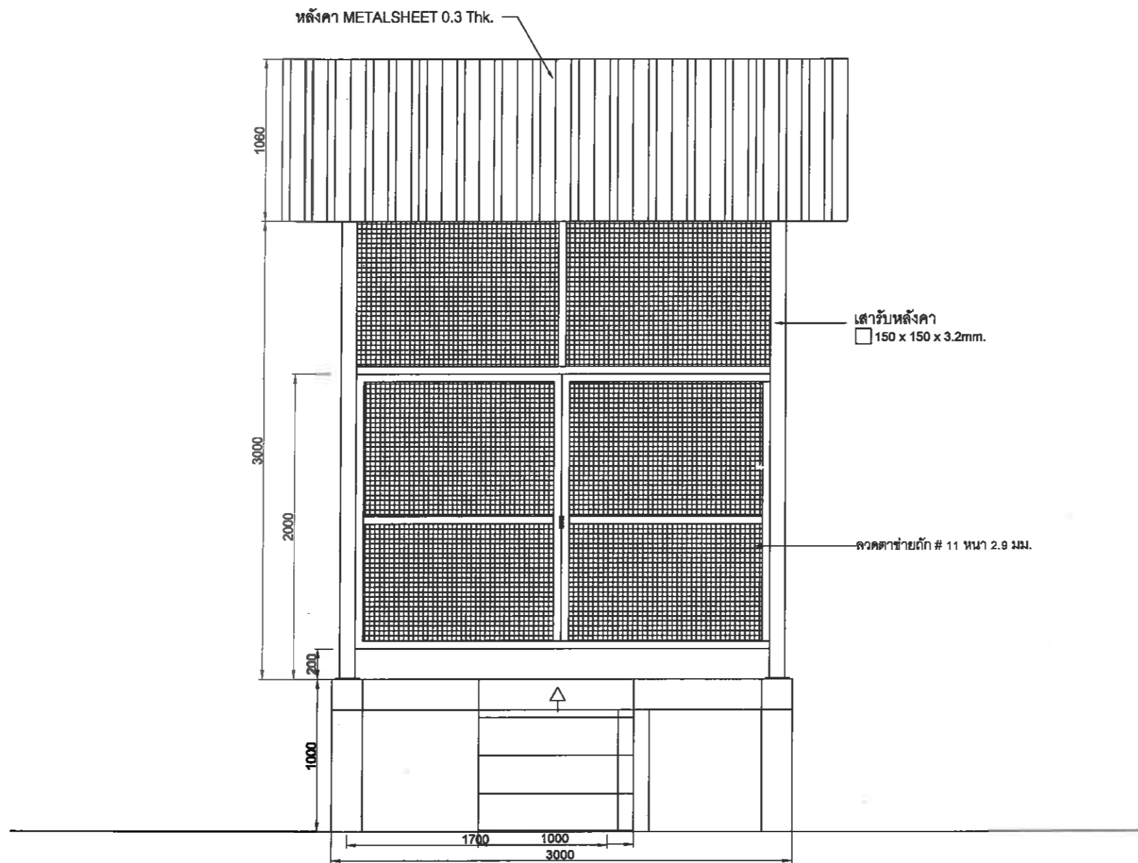
รูปด้าน E - E
