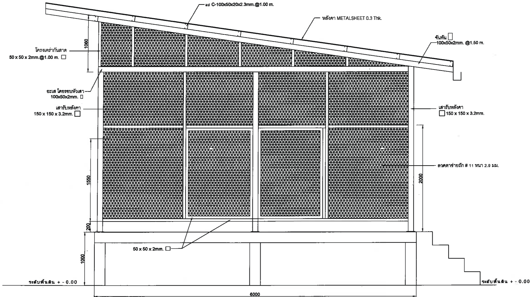
รูปด้าน D - D
