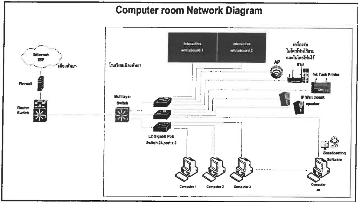
รูปที่ 1 แบบจำลองโครงสร้างการต่อเชื่อมเครือข่ายเน็ตเวิร์กภายในห้องปฏิบัติการคอมพิวเตอร์ โรงเรียนเมืองพัทยา 1-11
