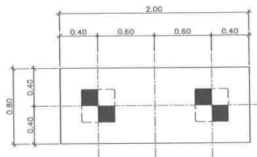
แปลน ฐานราก F2 มาตราส่วน 1 : 20
