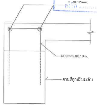
การเสริมหลังคาน T < 10 cm.
