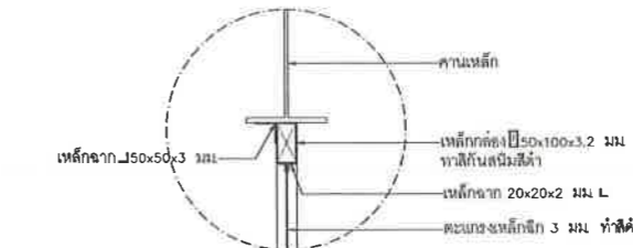
แบบขยาย B" มาตราส่วน 1:25
