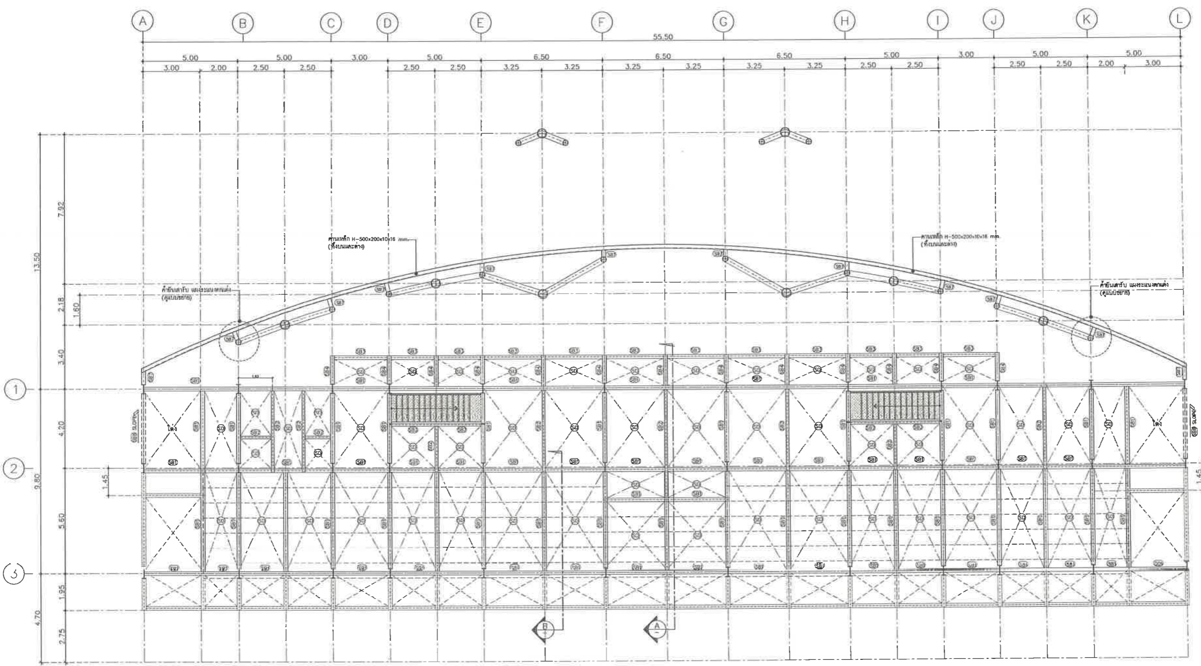
แปลนโครงสร้าง ชั้นที่ 2 มาตราส่วน 1:100
