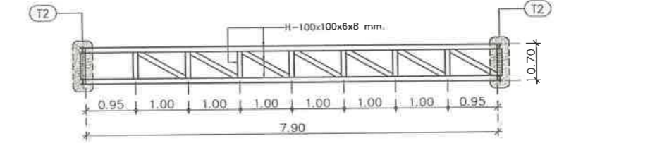
TRUSS T1A มาตราส่วน 1:50
