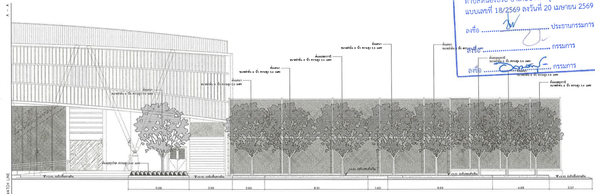
แบบขยาย รูปด้าน 2 (MATCH LINE A-A) มาตราส่วน 1 : 75
