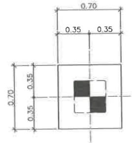
แปลน ฐานราก F1A มาตราส่วน 1 : 20
