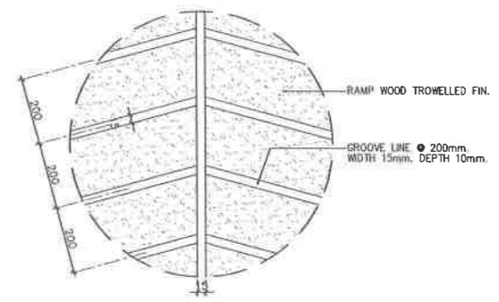
แบบขยายเซาะร่องพื้นทางลาด มาตราส่วน 1:25
