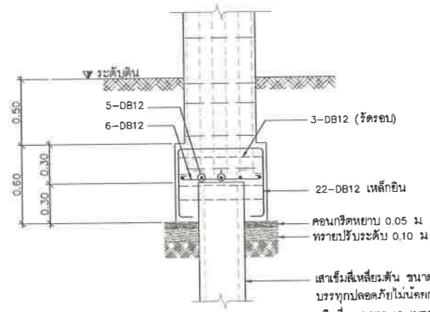
รูปตัด ฐานราก F1A มาตราส่วน 1 : 20
