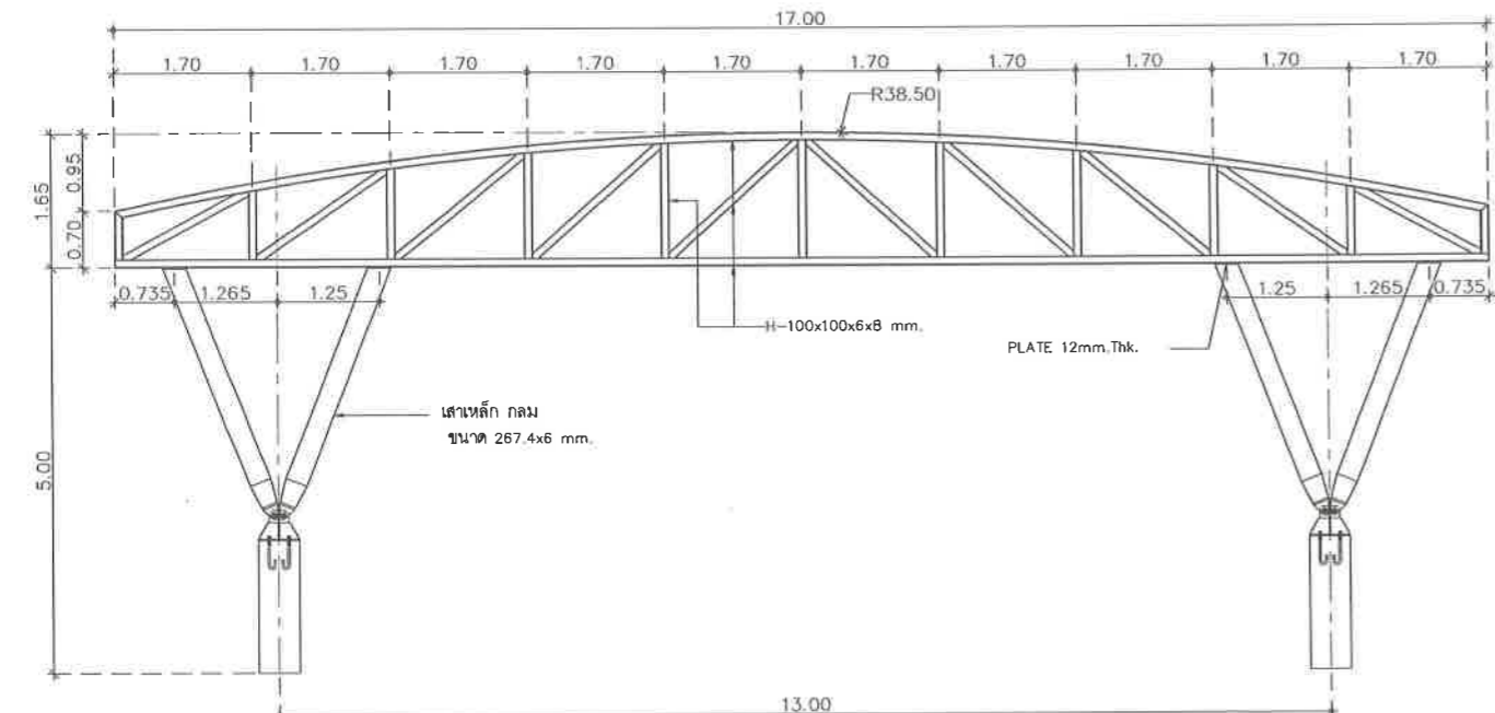
TRUSS T2 มาตราส่วน 1:50
