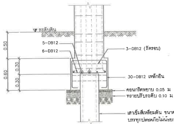
รูปตัด ฐานราก F1 มาตราส่วน 1 : 20
