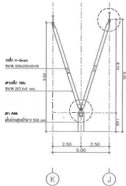
แบบขยายเสารับแฉ่งระแนงตกแต่ง 1A มาตราส่วน 1:100
