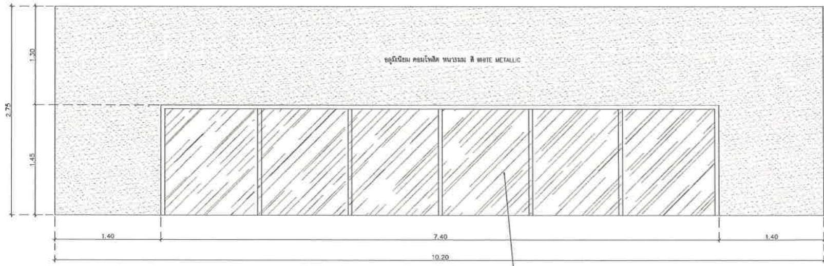
แปลนที่นั่งผู้พิการ มาตราส่วน 1:25
