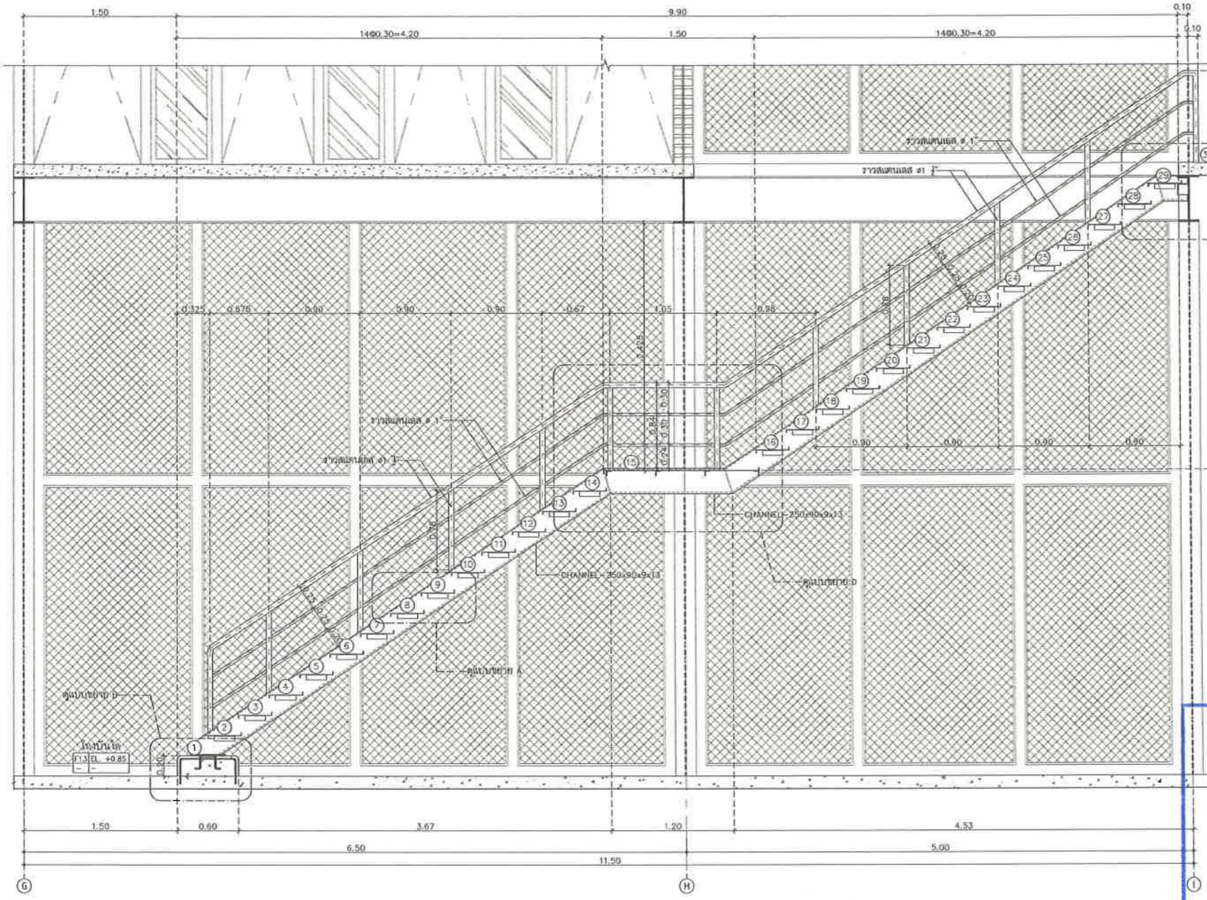
รูปตัดบันได มาตราส่วน 1:25
