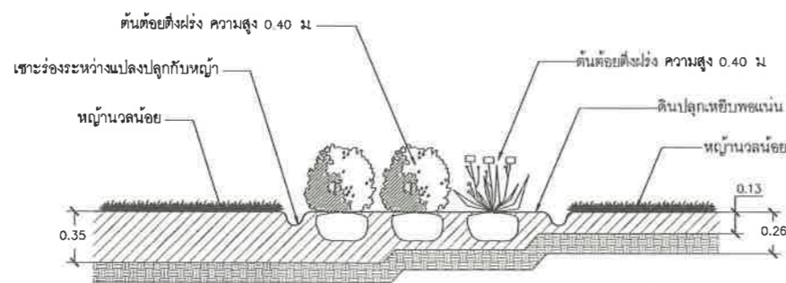
รูปตัดขยายการปลูกไม้พุ่มและหญ้า มาตราส่วน NTS
