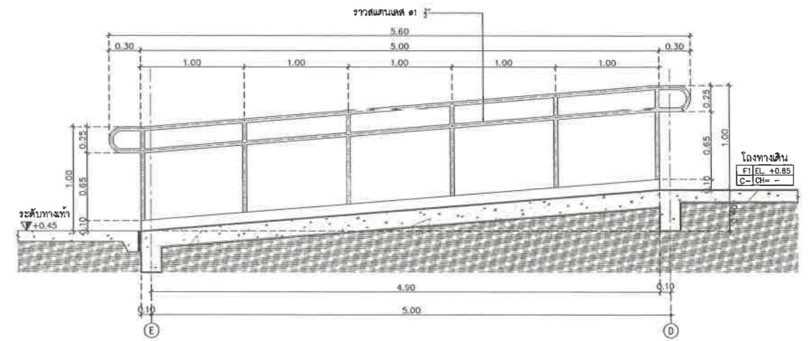
รูปตัด B มาตราส่วน 1:25
