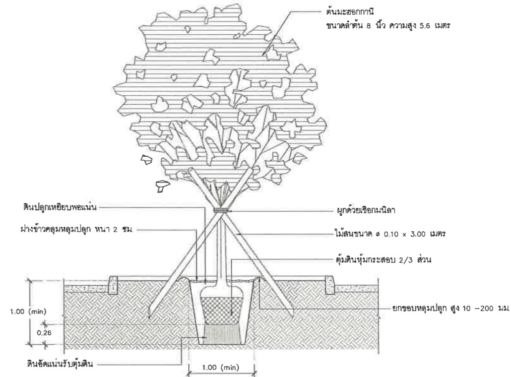
รูปตัดพันธุ์ไม้ชนิดที่ 2 มาตราส่วน 1 : 40
