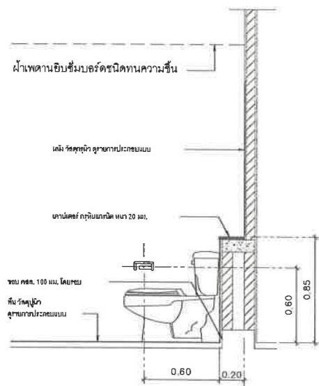
แบบการติดตั้งอุปกรณ์ห้องส่วนนั่งราบ
