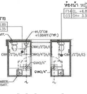
แบบน้ำดีห้องน้ำชาย ห้องอาบน้ำ มาตราส่วน 1:50
