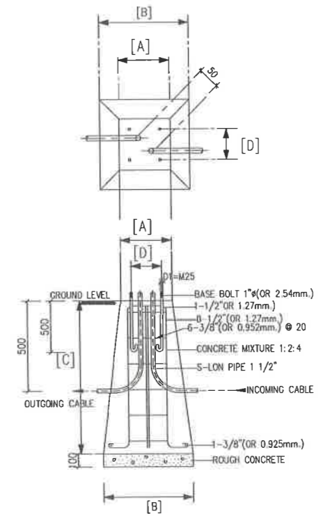
รูปขยายแสดงฐานโคมไฟ
