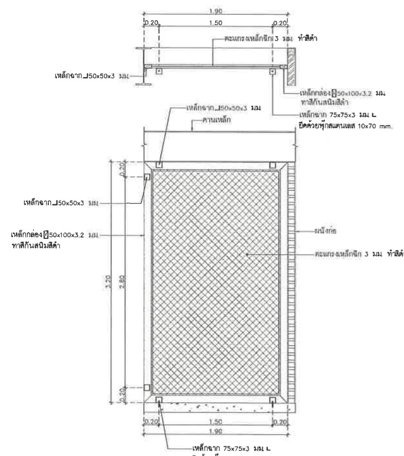
แบบขยายตะแกรงเหล็กฉีก มาตราส่วน 1:25
