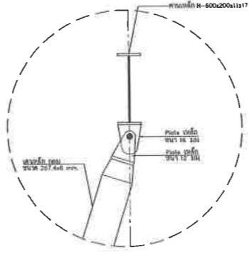
แบบขยายหัวเสารับแฉงระแนงตกแต่ง มาตราส่วน NTS
