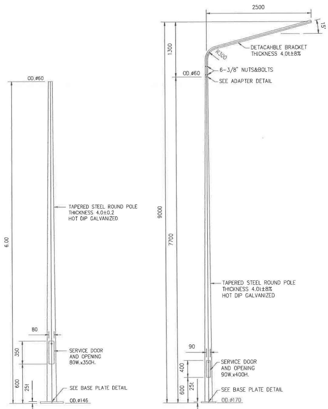
แบบ DETAIL เสาไฟแสงสว่างภายนอก มาตรฐาน NTS.
