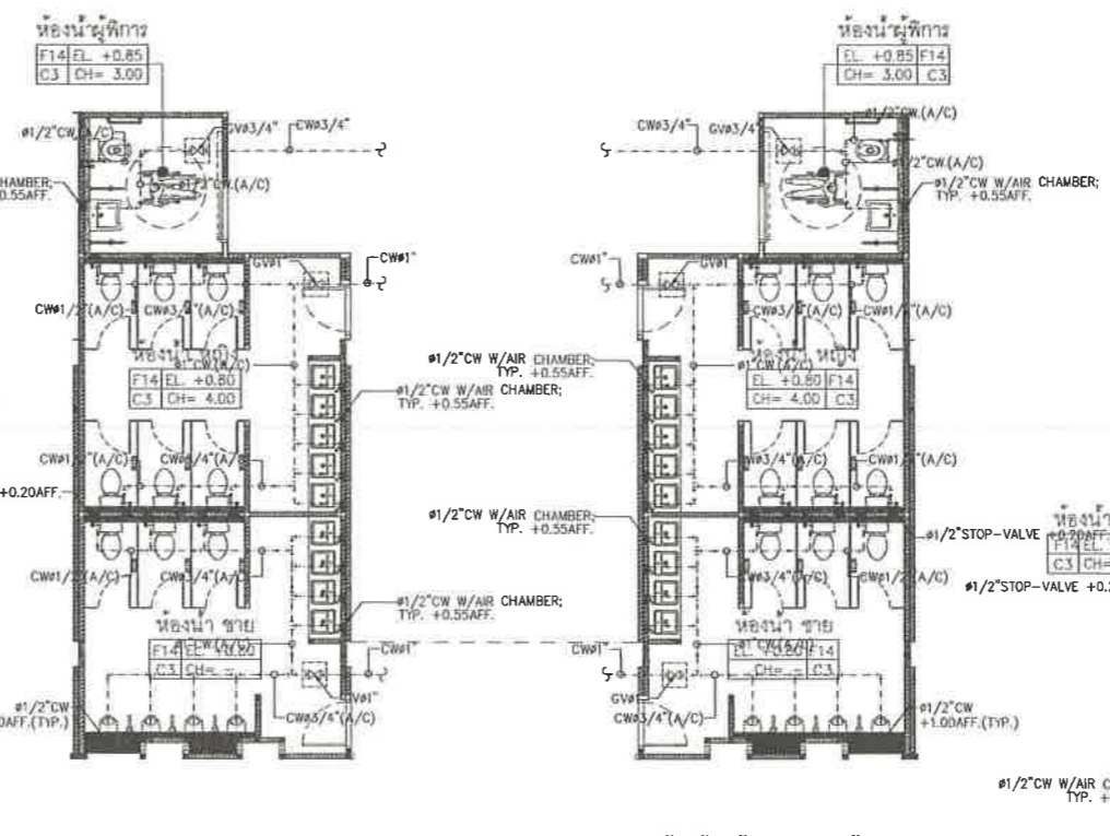
แบบน้ำดีห้องน้ำชาย ห้องผู้ฝึกการ 1 มาตราส่วน 1:50
