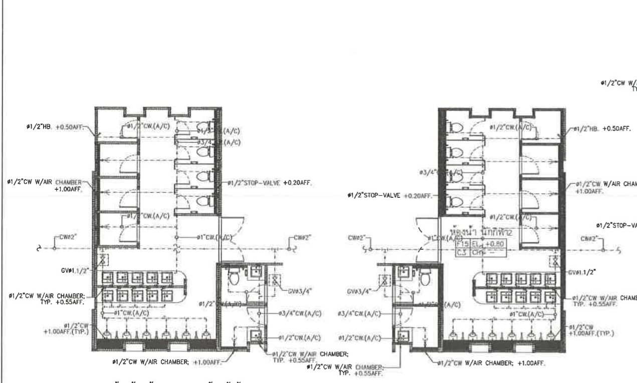
แบบน้ำดีห้องน้ำนักกีฬา 1, ห้องน้ำผู้ตัดสิน มาตราส่วน 1:50
