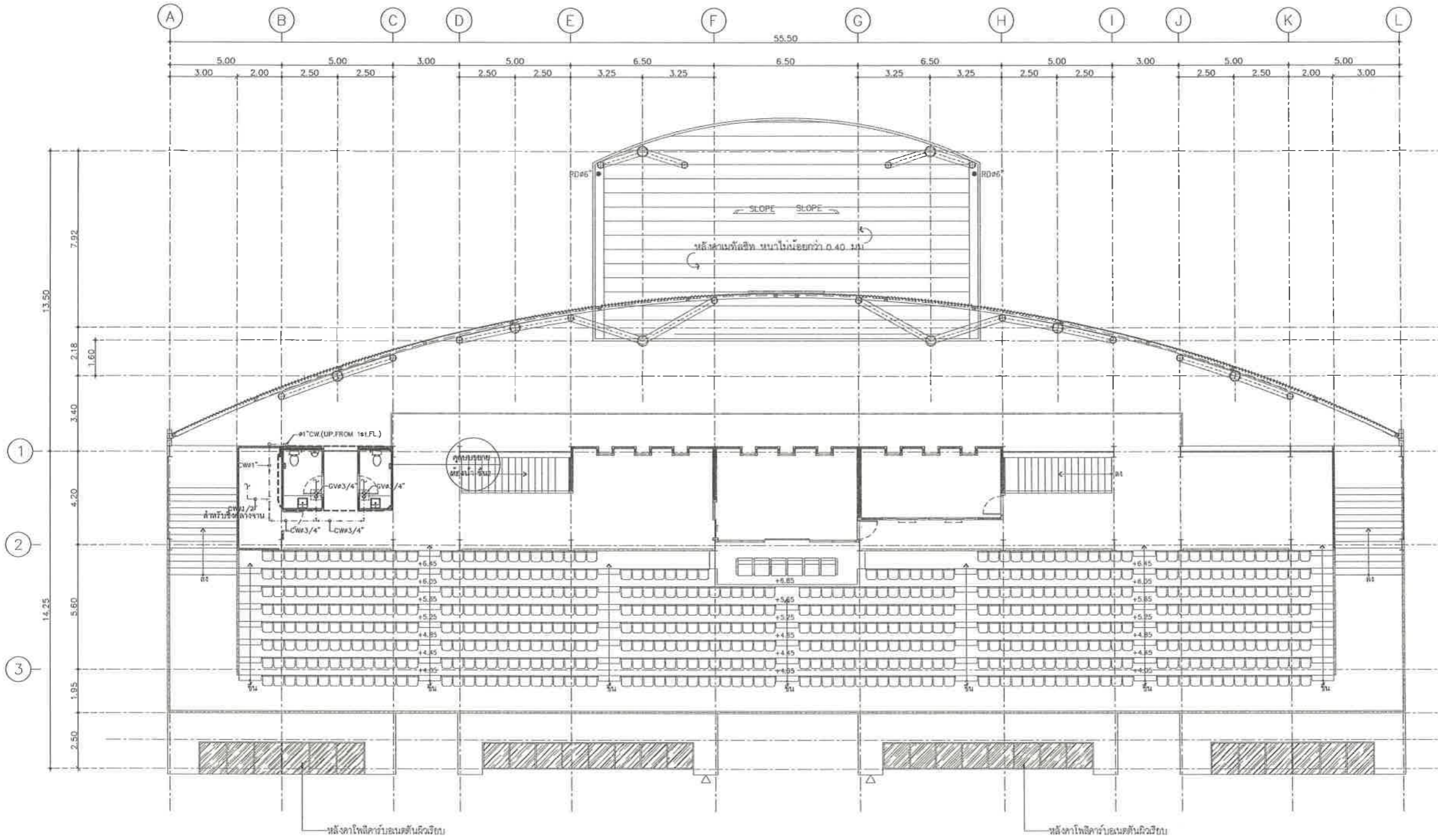
แบบระบบน้ำดีอิมจันทร์ ชั้น 2 มาตราส่วน 1:100
