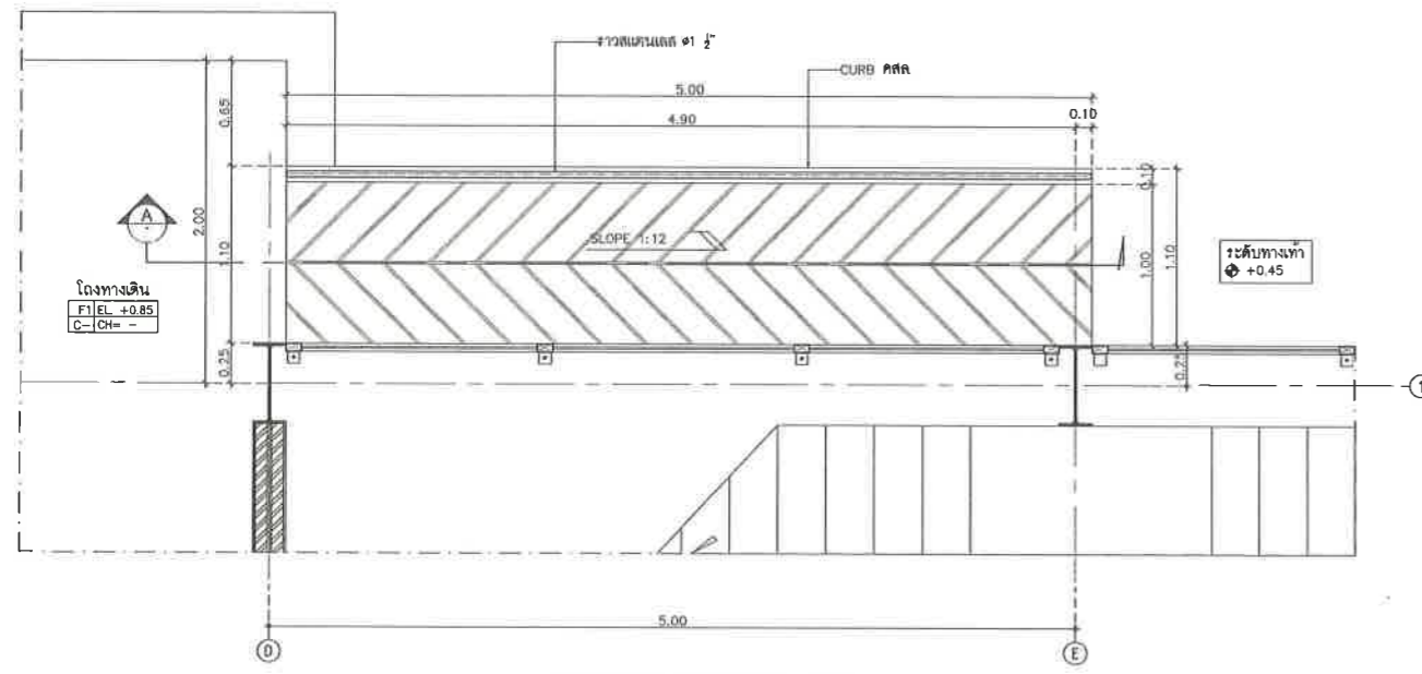
แบบขยายทางลาดคนพิการ 3B มาตราส่วน 1:25
