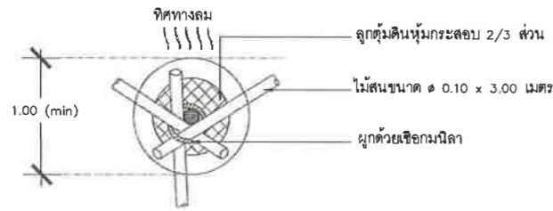
แปลนพันธุ์ไม้ชนิดที่ 1 มาตราส่วน 1 : 40
