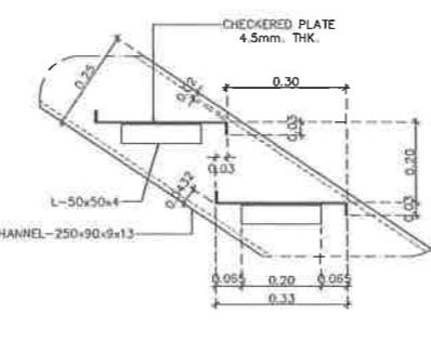
แบบขยาย A มาตราส่วน 1:25
