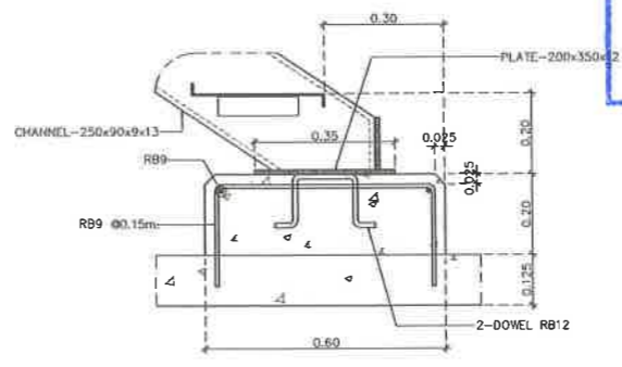
แบบขยาย B มาตราส่วน 1:25
