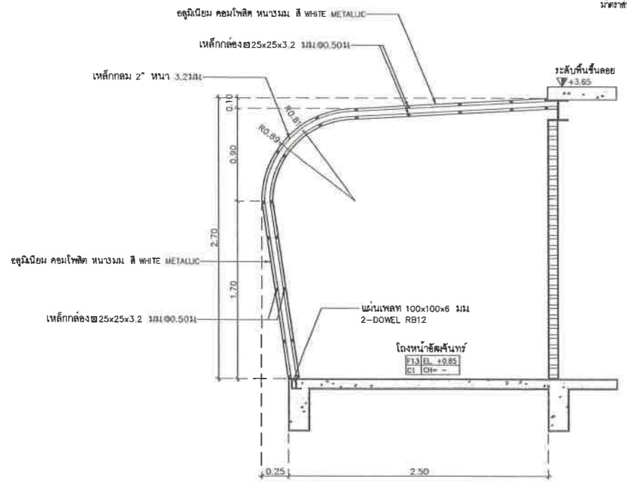
รูปตัด A มาตราส่วน 1:25
