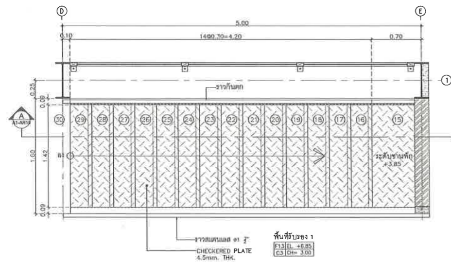
แปลนขยายบันได ST 2B ชั้นที่ 2 มาตราส่วน 1:25
