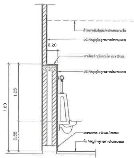
แบบการติดตั้งโถปัสสาวะ
