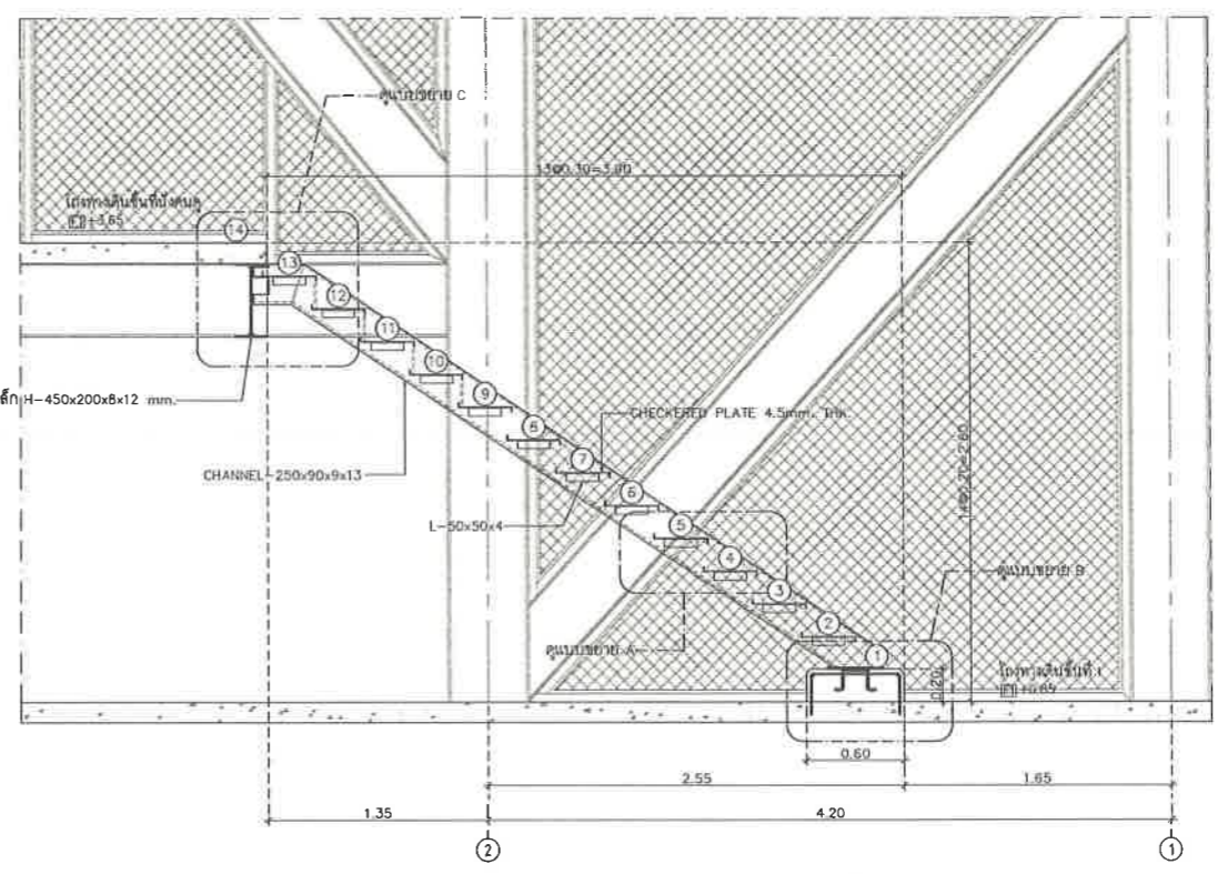
รูปตัดบันได B มาตราส่วน 1:25
