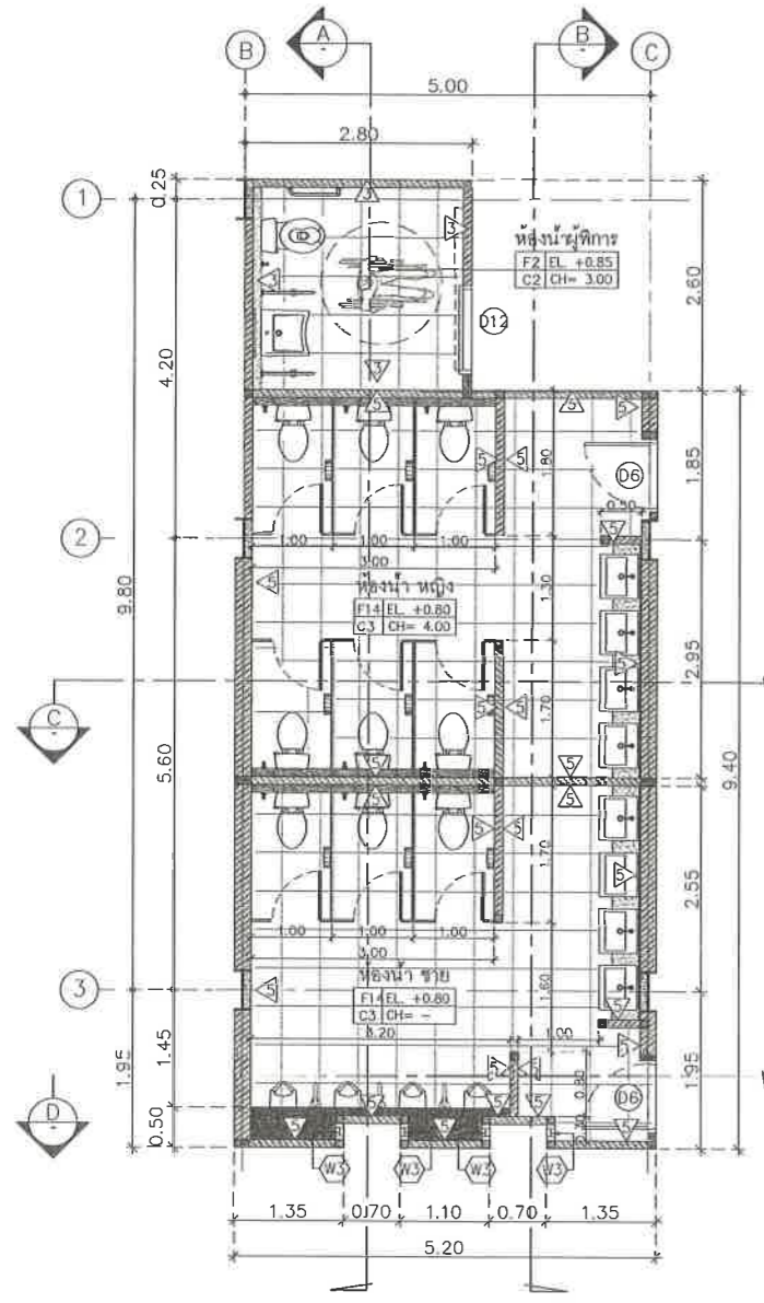
แปลนขยายห้องน้ำ ชาย, หญิง, ผู้พิการ มาตราส่วน 1 : 50
