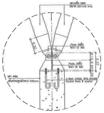
แบบขยายฐานเสารับแฉงระแนงตกแต่ง มาตราส่วน NTS
