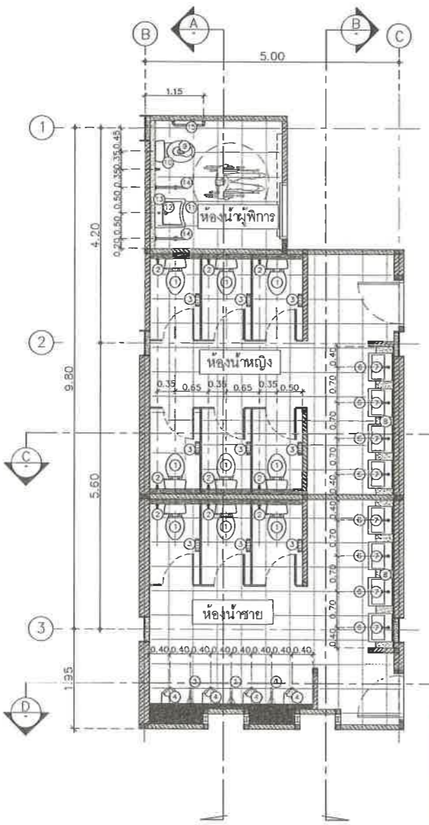
แปลนแสดงรายละเอียดสุขภัณฑ์ ชาย, หญิง, ผู้พิการ มาตราส่วน 1 : 50
