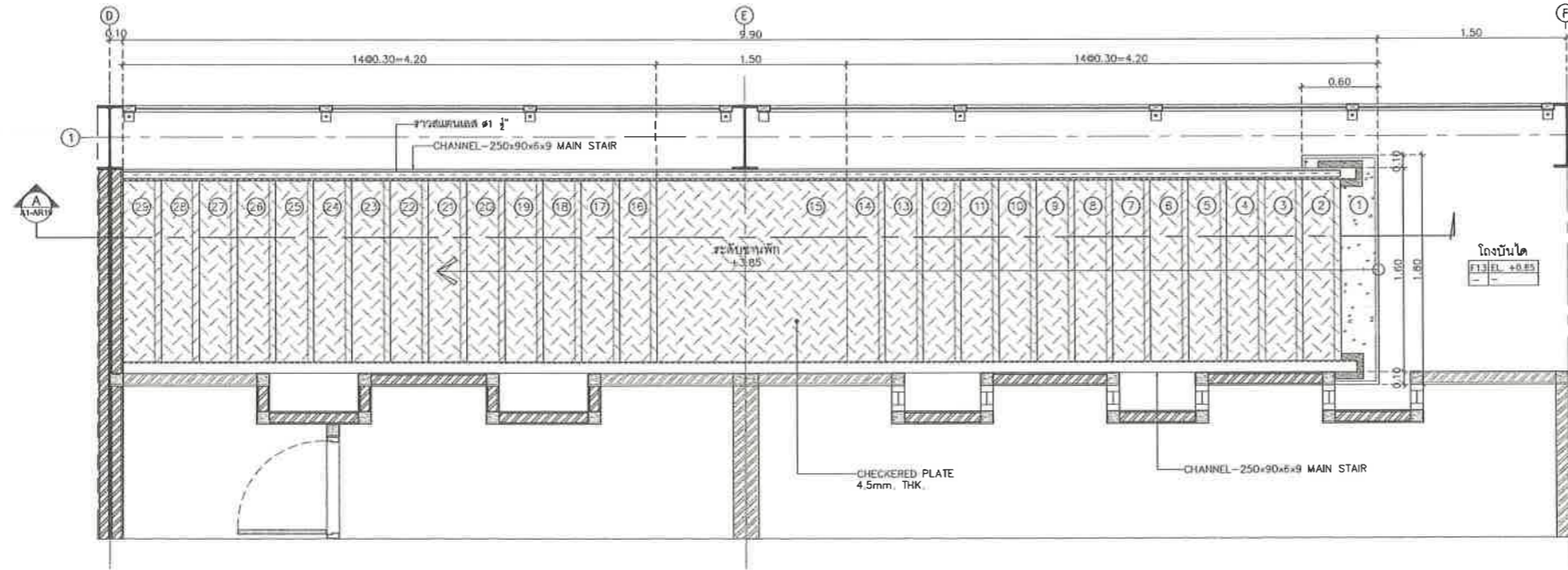
แปลนขยายบันได ST 2B ชั้นที่ 1 มาตราส่วน 1:25
