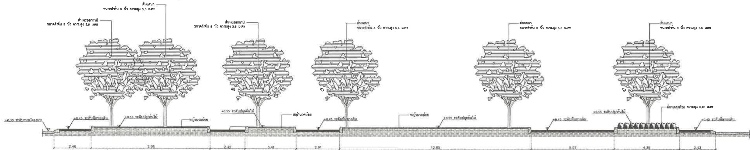
แบบขยาย รูปตัด G-G มาตราส่วน 1 : 75
