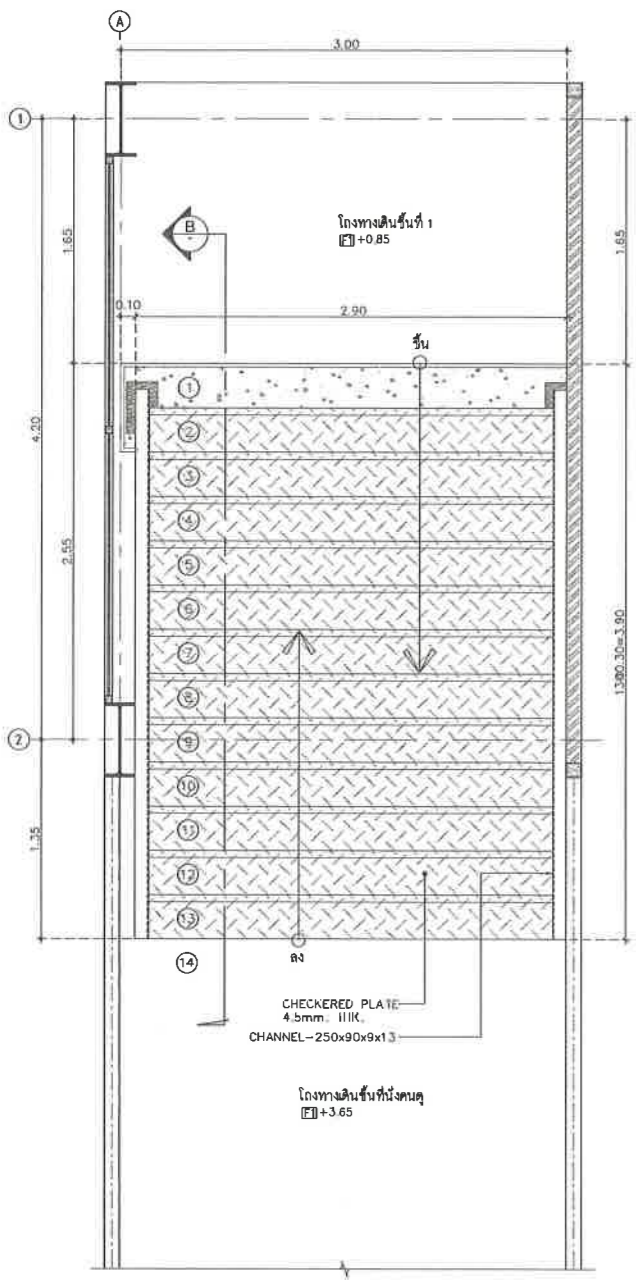
แปลนขยายบันได ST มาตราส่วน 1:25
