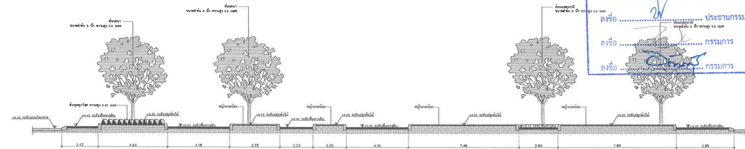
แบบขยาย รูปตัด H-H มาตราส่วน 1 : 75
