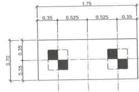
แปลน ฐานราก F2A มาตราส่วน 1 : 20
