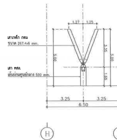
แบบขยายเสารับ Canopy 1A มาตราส่วน 1:100
