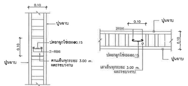
รายละเอียดหน้าตัดคานยื่นคานยื่นทุกระยะ 3.00 m. แนวตั้งและรอบวง
