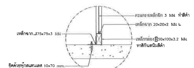
แบบขยาย A" มาตราส่วน 1:25
