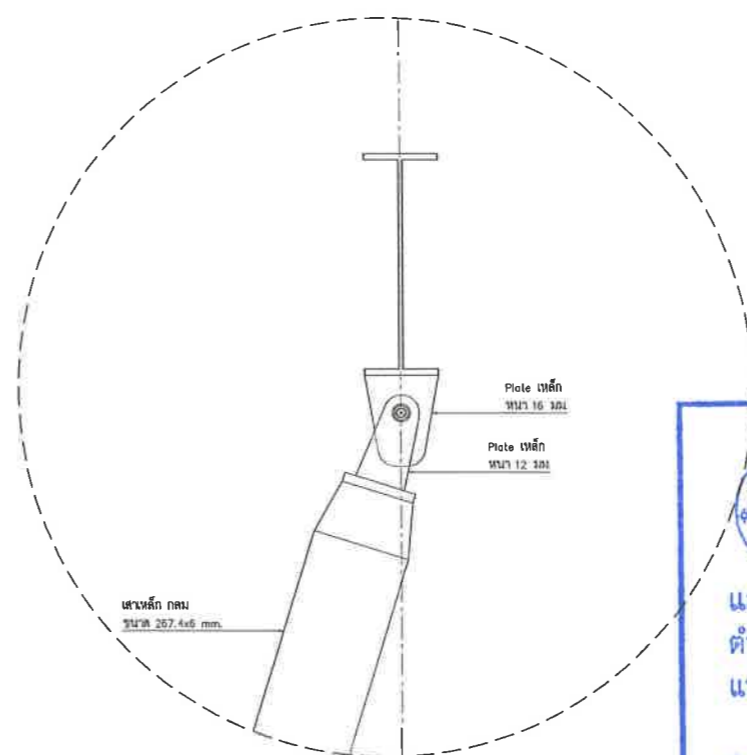
แบบขยายหัวเสารับแฉ่งระแนงตกแต่ง มาตราส่วน 1:10
