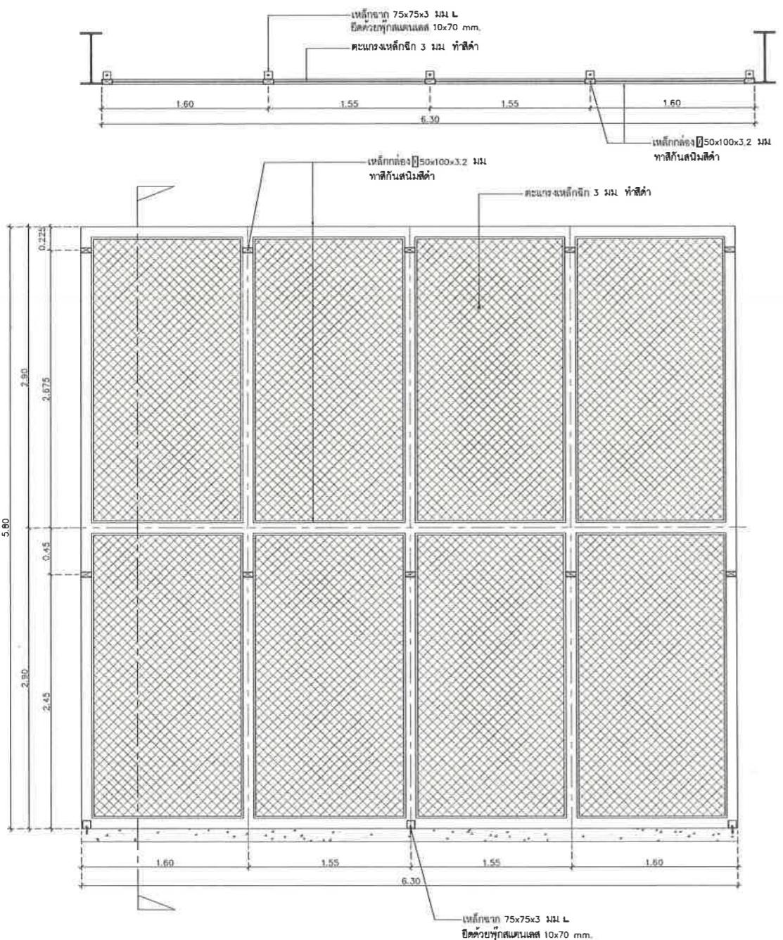
แบบขยายแผงตะแกรงเหล็กฉีก 05 มาตราส่วน 1:25
