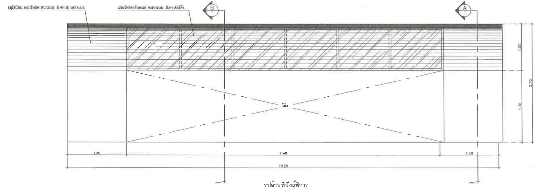
รูปด้านที่นั่งผู้พิการ มาตราส่วน 1:25
