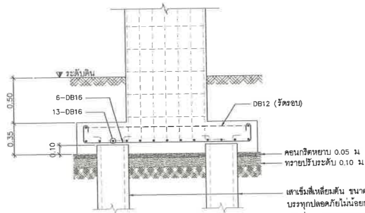
รูปตัด ฐานราก F2 มาตราส่วน 1 : 20
