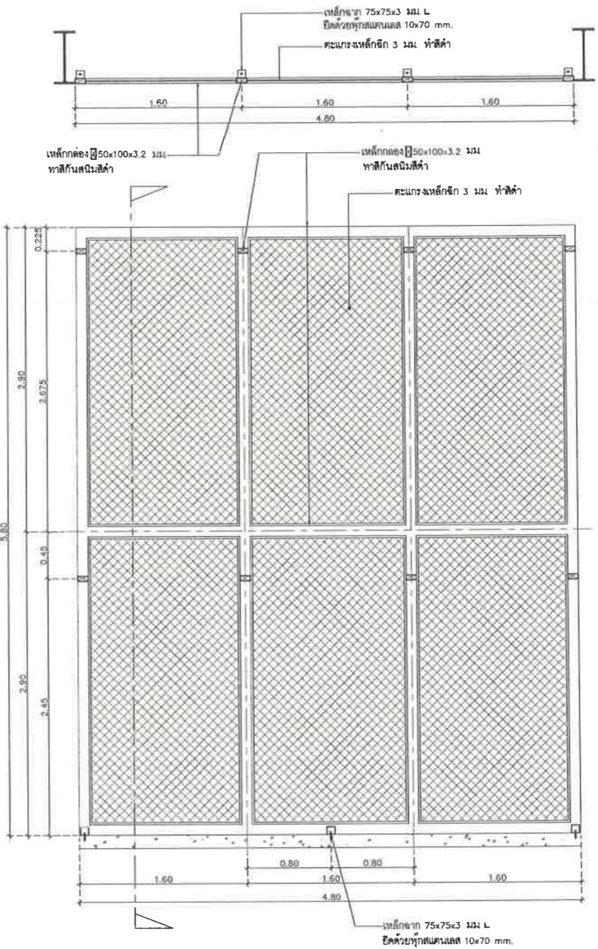
แบบขยายแผงตะแกรงเหล็กฉีก 06 มาตราส่วน 1:25
