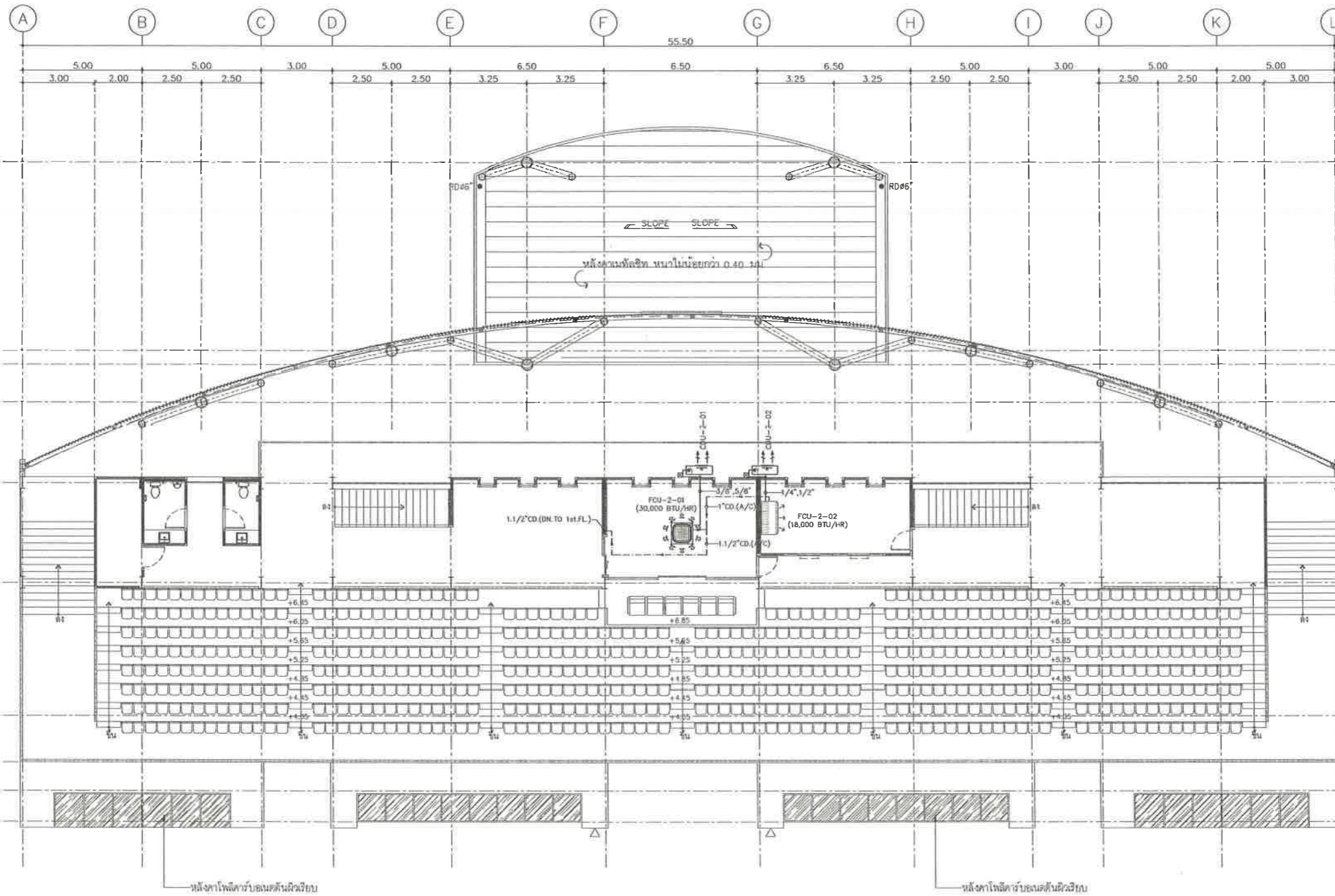
แบบระบบเครื่องปรับอากาศ ชั้น 2 มาตราส่วน 1:100
