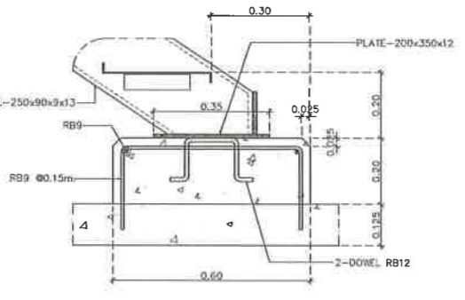
แบบขยาย B มาตราส่วน 1:25
