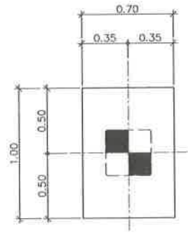
แปลน ฐานราก F1 มาตราส่วน 1 : 20
