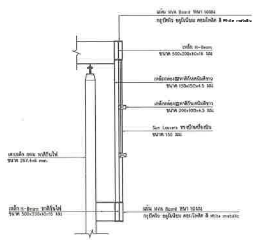
ขยายค้ำยันเสารับ แฉงระแนงตกแต่ง มาตราส่วน NTS
