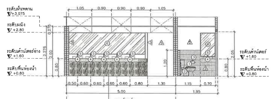
รูปตัด E มาตราส่วน 1 : 50
