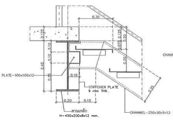
แบบขยาย C มาตราส่วน 1:25
