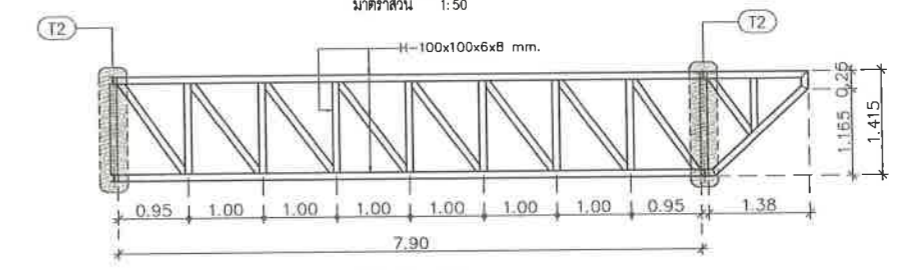
TRUSS T1B มาตราส่วน 1:50
