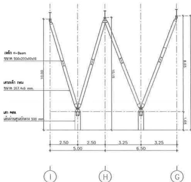
แบบขยายเสารับแฉ่งระแนงตกแต่ง 2A มาตราส่วน 1:100
