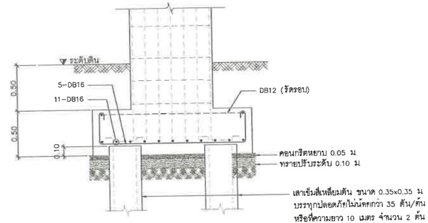
รูปตัด ฐานราก F2A มาตราส่วน 1 : 20
