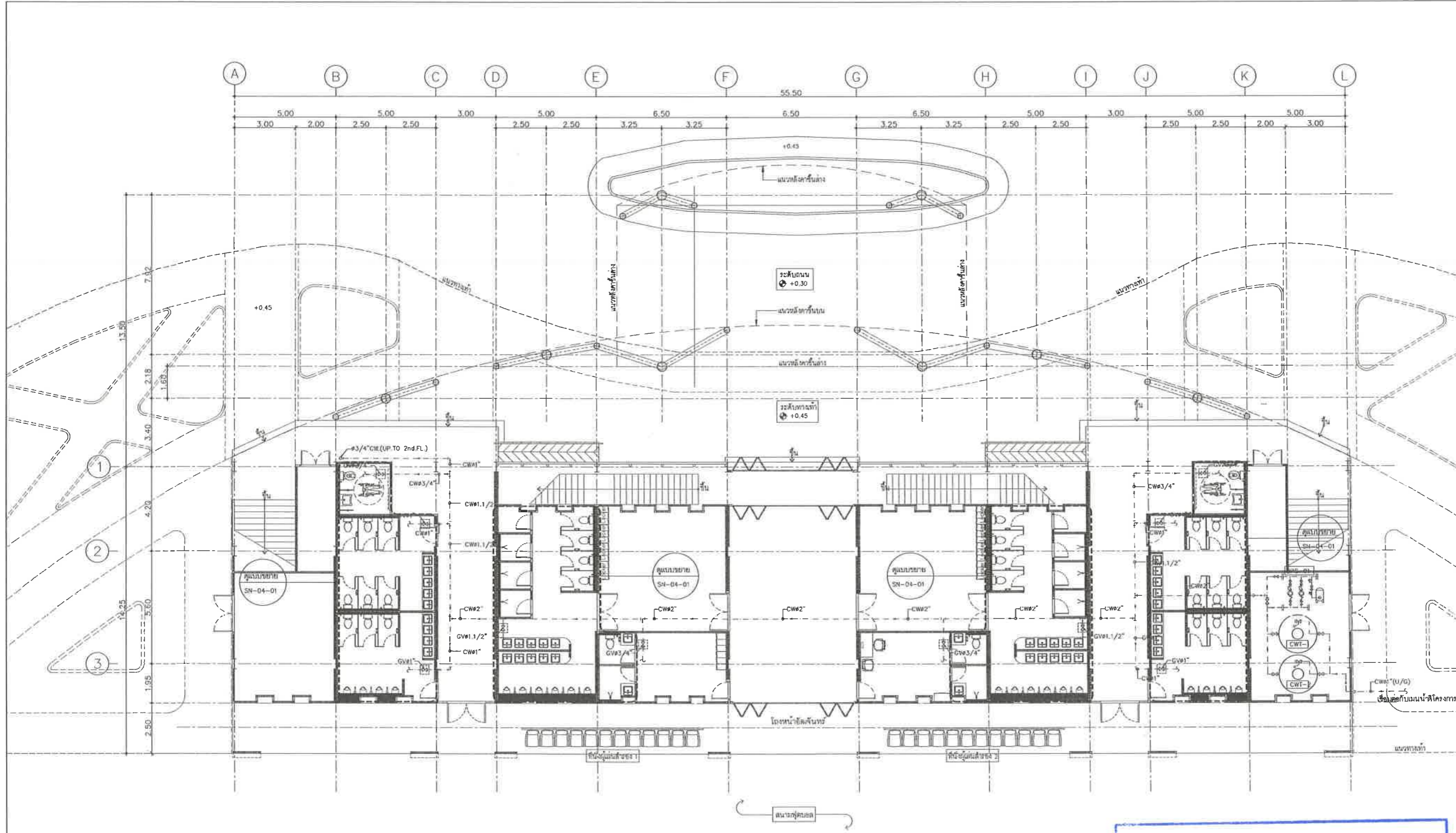
แบบระบบน้ำดีอิมโชนท์ ชั้น 1 มาตราส่วน 1:100
