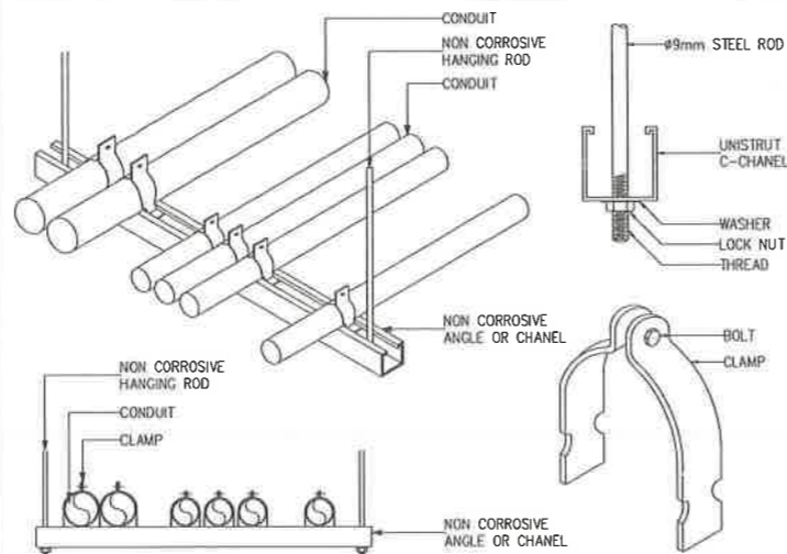
02 MULTIPLES CONDUIT SUPPORT NTS
