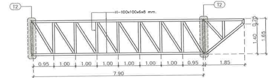
TRUSS T1C มาตราส่วน 1:50
