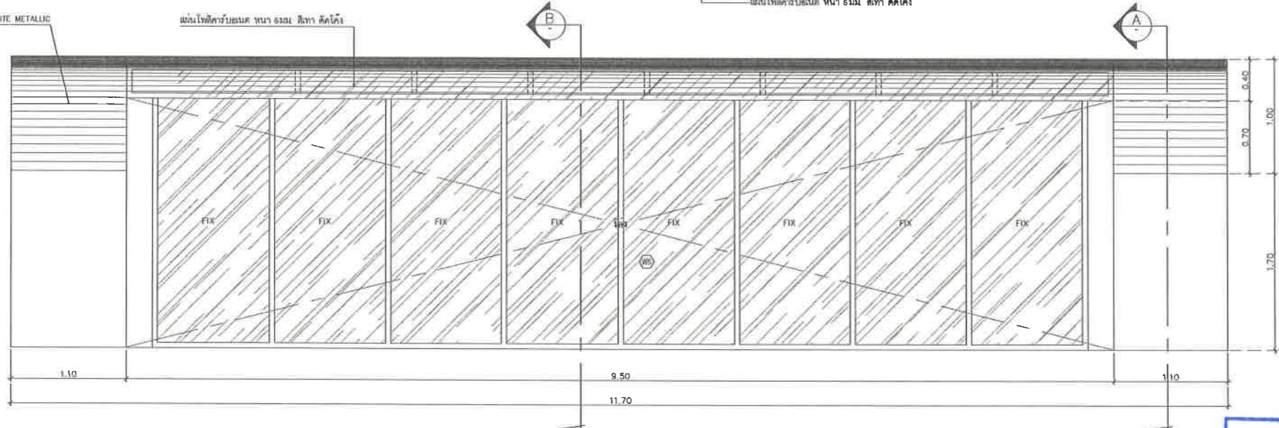
รูปด้านที่นั่งตัวสำรอง มาตราส่วน 1:25
