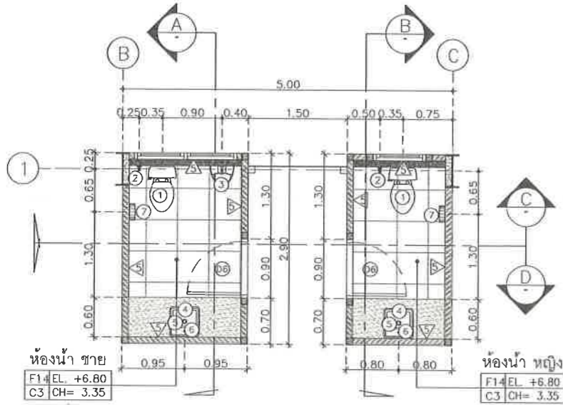
แปลนขยายห้องน้ำ ชาย, หญิง, ชั้นที่ 2 มาตราส่วน 1 : 50
