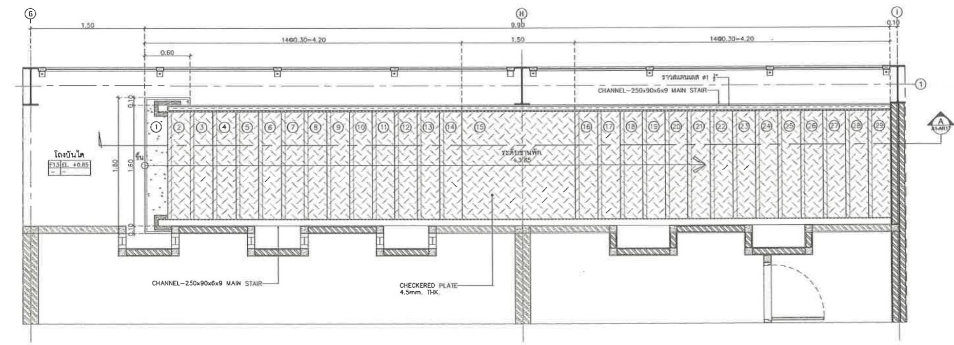
แปลนขยายบันได ST 2A ชั้นที่ 1 มาตราส่วน 1:25
