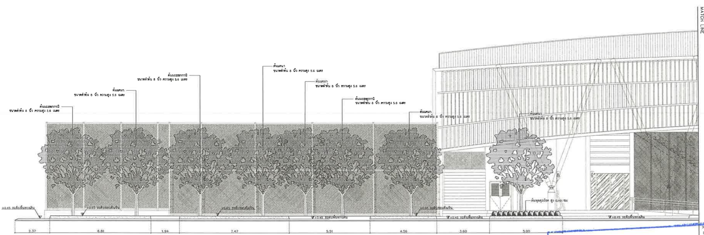
แบบขยาย รูปด้าน 1 (MATCH LINE A-A) มาตราส่วน 1 : 75
