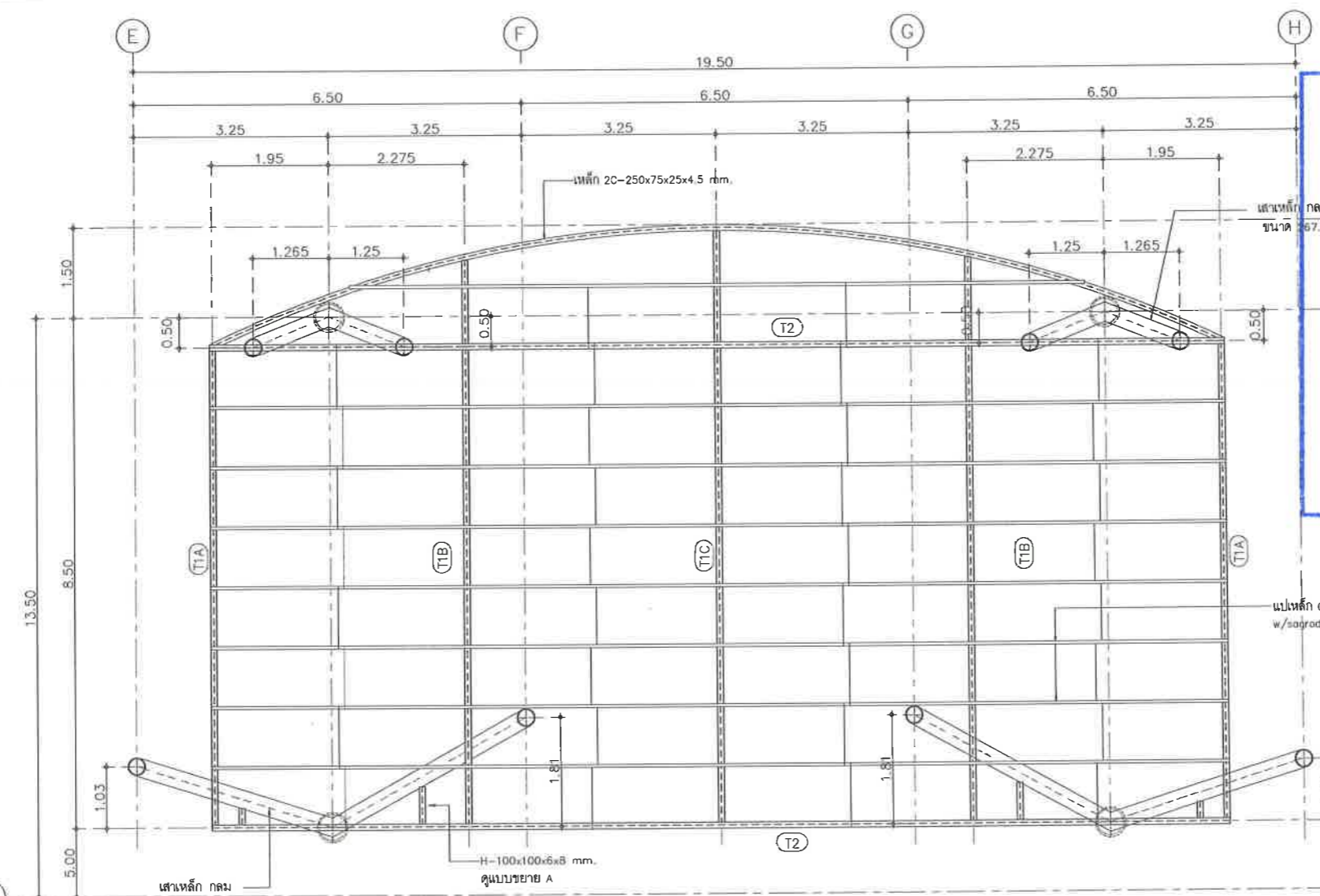
แปลนโครงสร้างหลังคา DROP OFF มาตราส่วน 1:50
