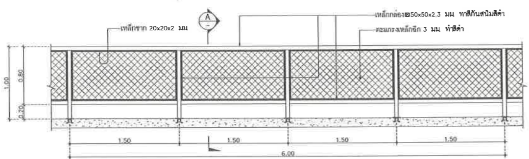
แบบขยาย A มาตราส่วน 1:25
