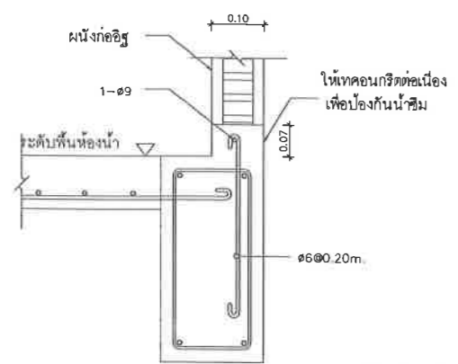
รายละเอียดการเทคอนกรีตและเสริมเหล็กบริเวณรอยต่อพื้นห้องน้ำเพื่อป้องกันน้ำซึม
