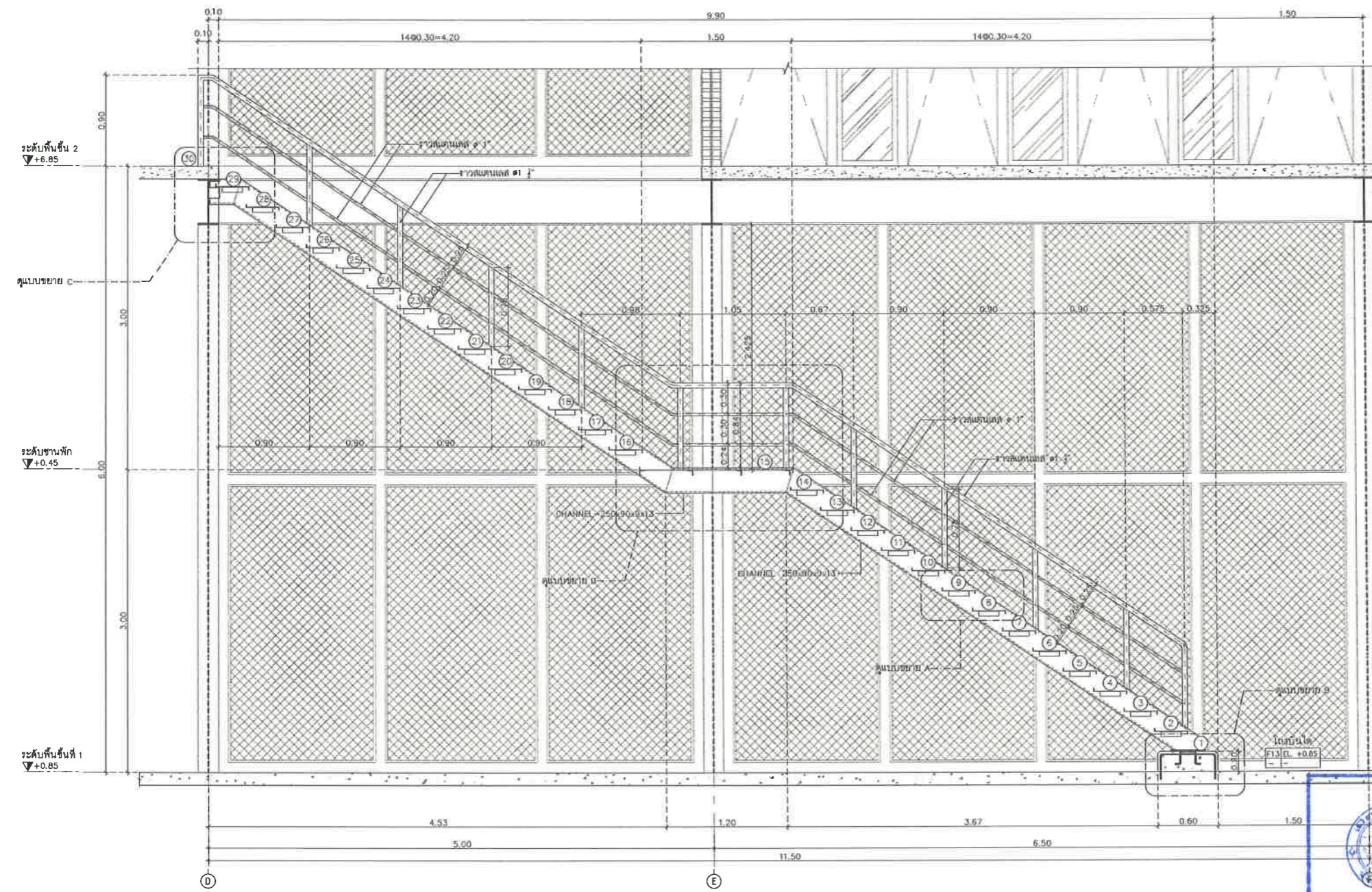
รูปตัดบันได มาตราส่วน 1:25
