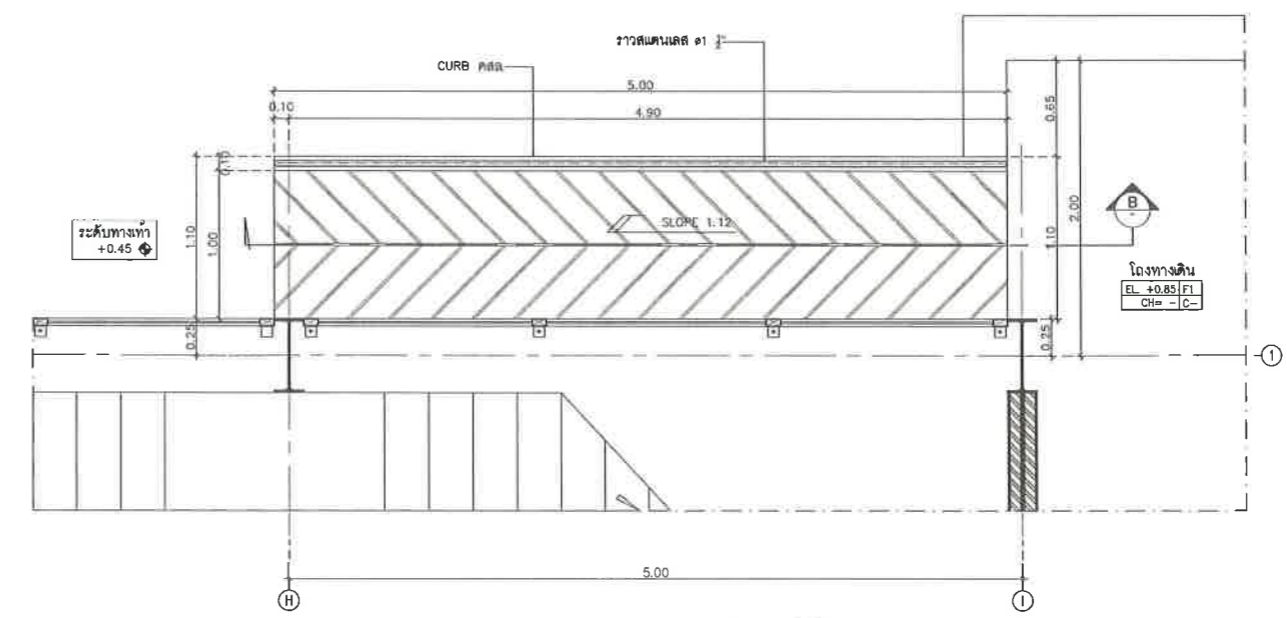
แบบขยายทางลาดคนพิการ 3A มาตราส่วน 1:25
