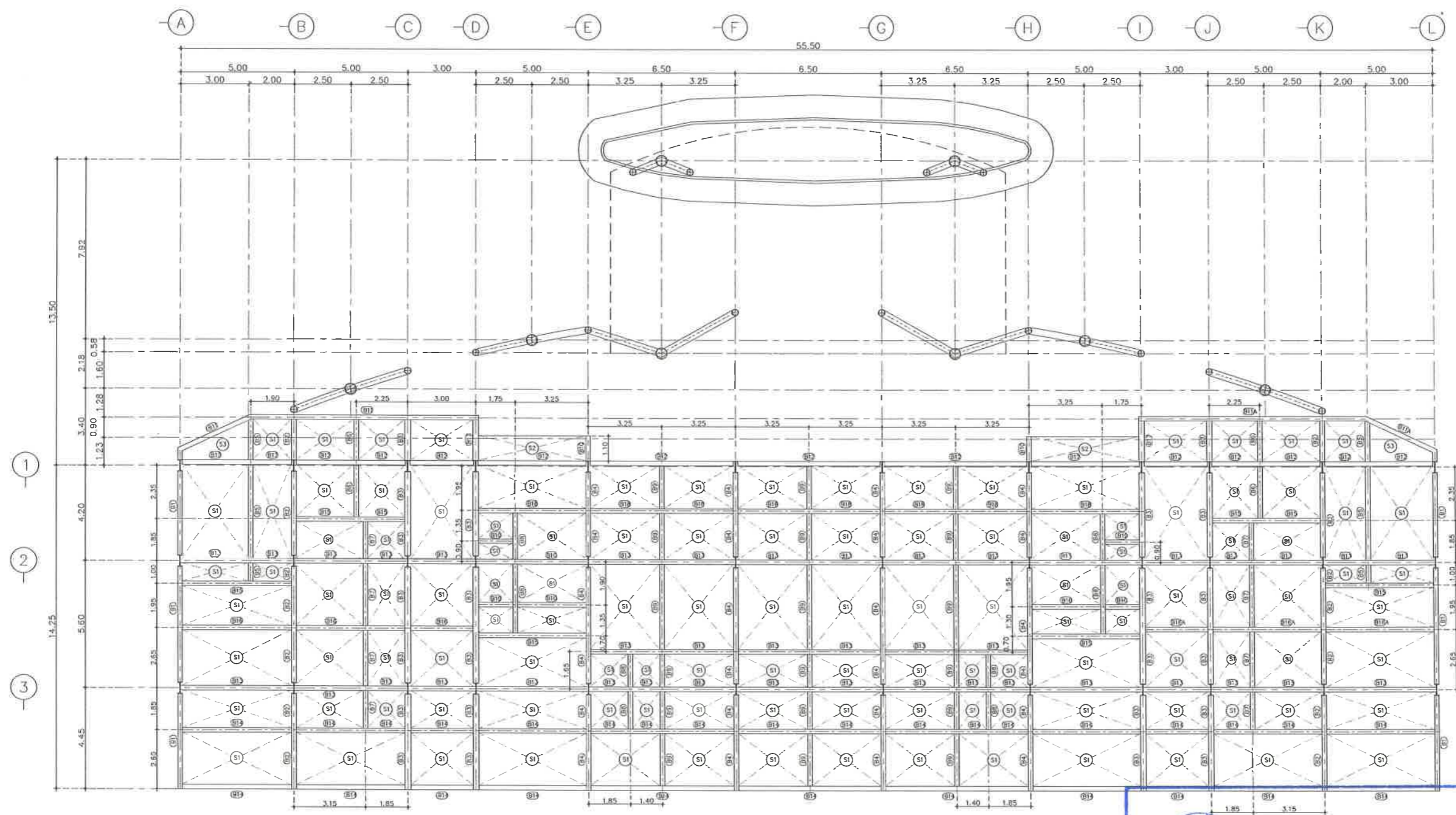
แปลนคาน,พื้น ชั้นที่ 1 มาตราส่วน 1:100
