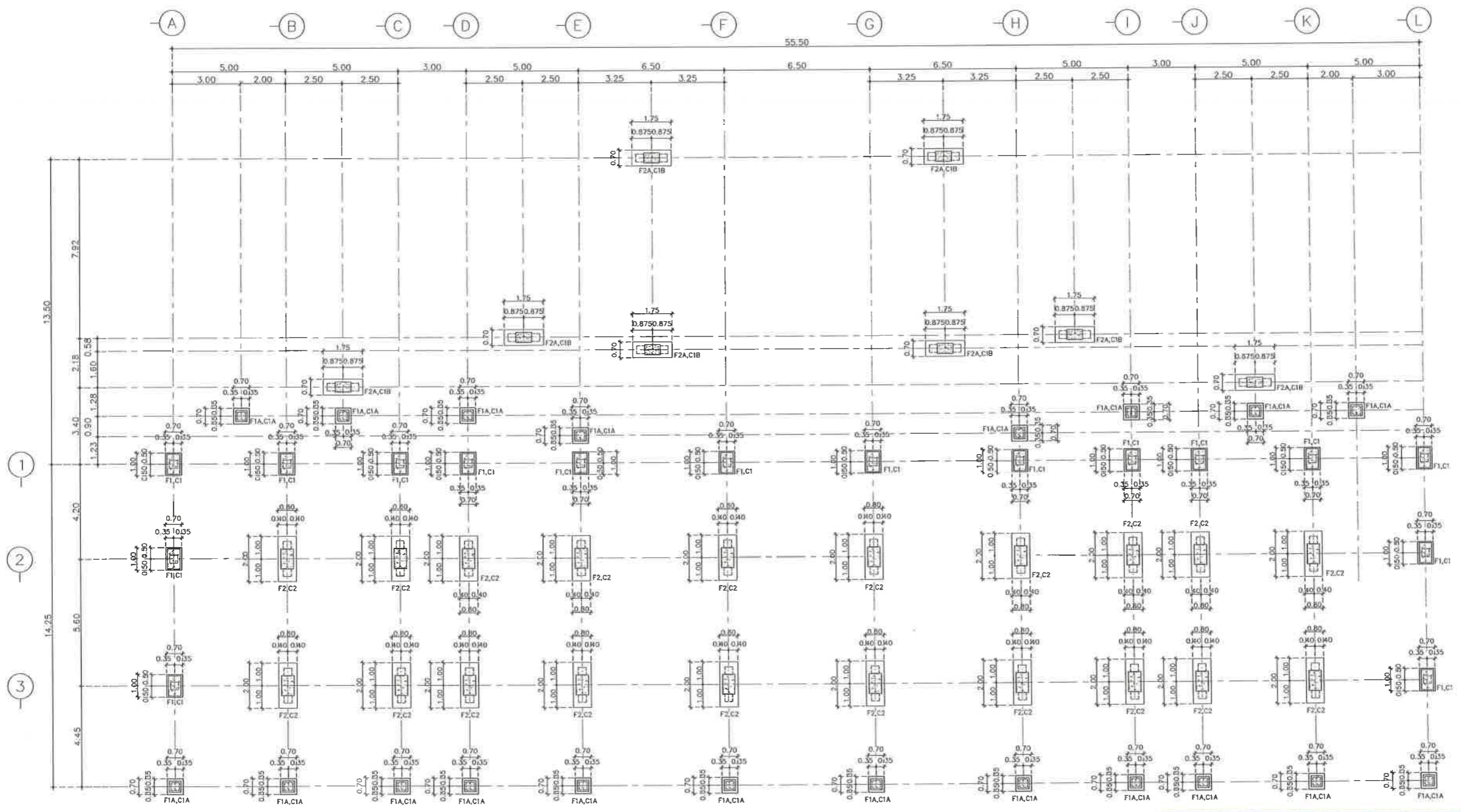
แปลนฐานราก,เสาตอม่อ มาตรฐาน 1 : 100
