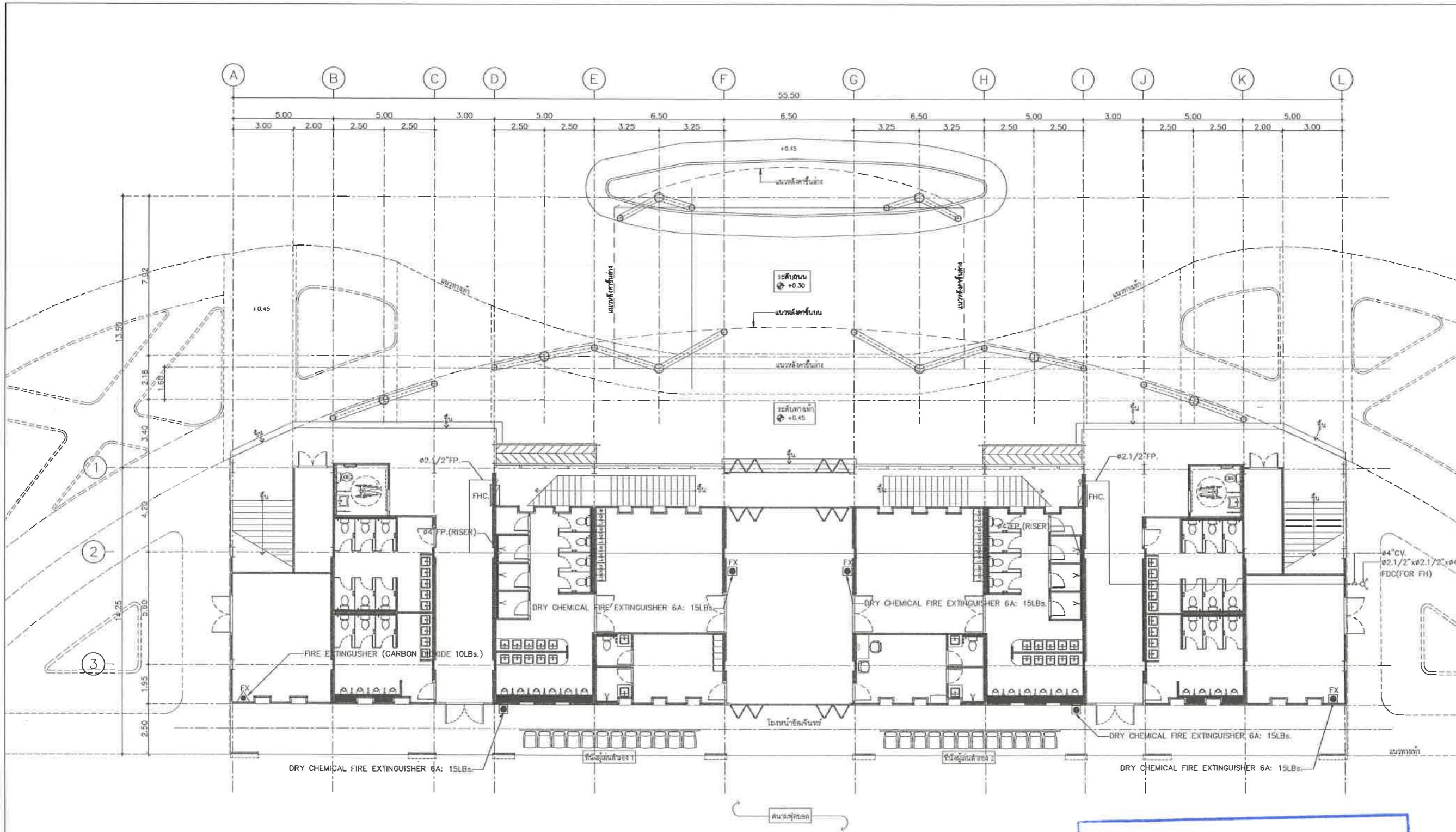
แบบระบบดับเพลิง ชั้น 1 มาตราส่วน 1:75
