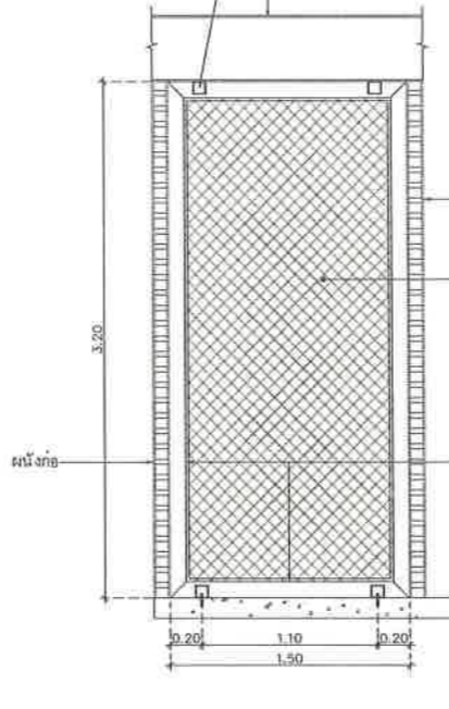
แบบขยายตะแกรงเหล็กฉีก มาตราส่วน 1:25
