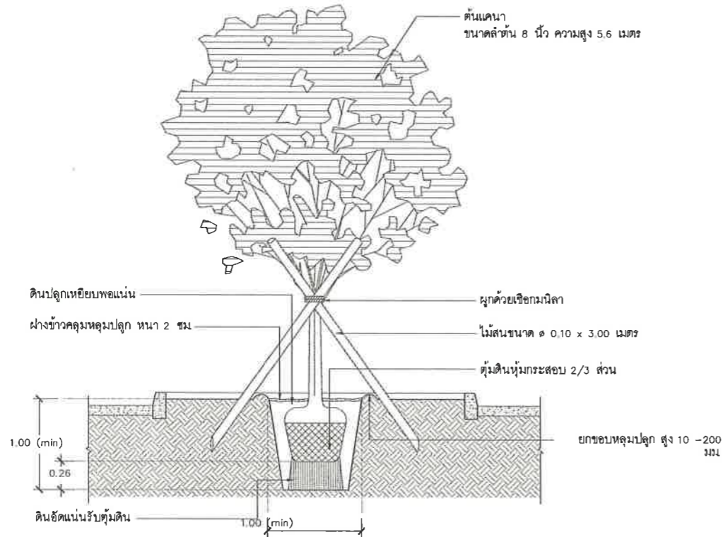
รูปตัดพันธุ์ไม้ชนิดที่ 1 มาตราส่วน 1 : 40
