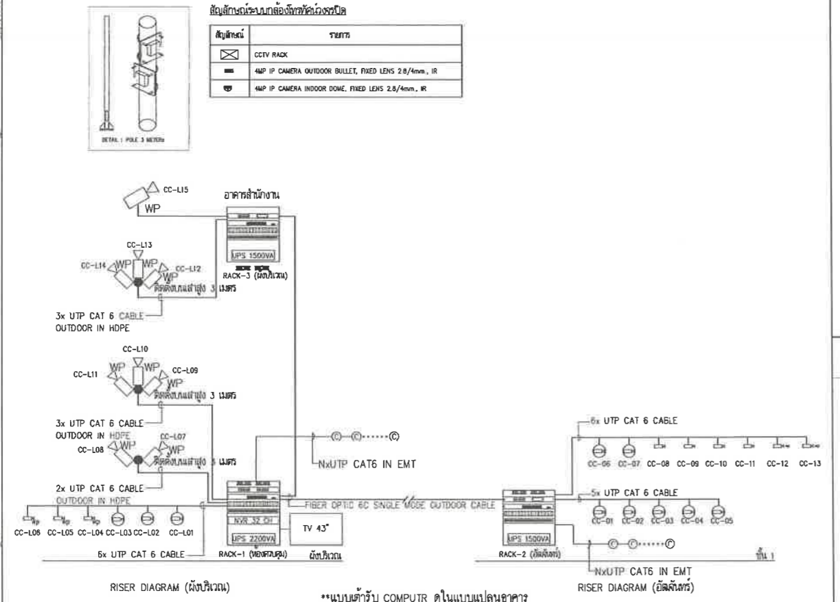
ระบบกล้องวงจรปิด RISER DIAGRAM มาตรฐาน NTS.
