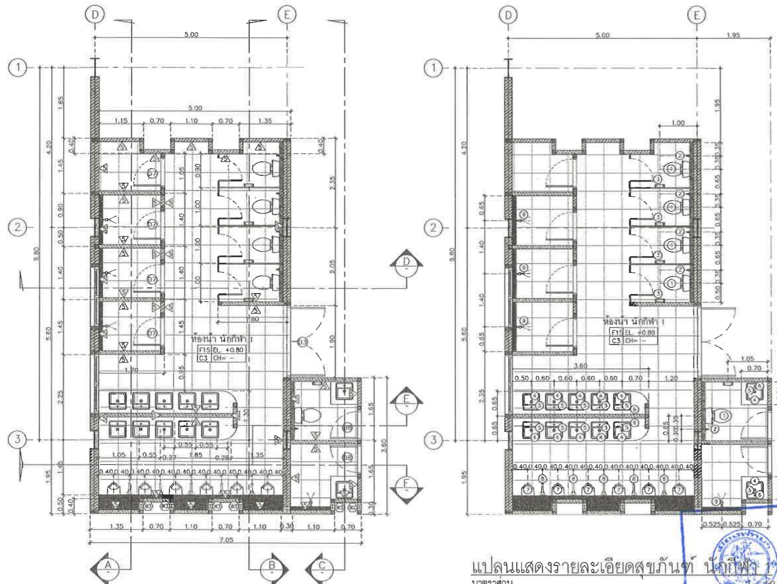
แปลนขยายห้องน้ำ นักกีฬา 1 มาตราส่วน 1 : 50
