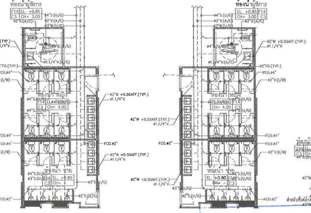
แบบน้ำดีห้องน้ำชาย ห้องผู้ฝึกการ 1 มาตราส่วน 1:50
