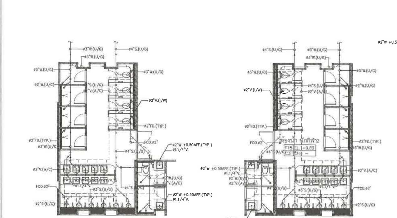
แบบน้ำดีห้องน้ำนักกีฬา 1, ห้องน้ำผู้ตัดสิน มาตราส่วน 1:50
