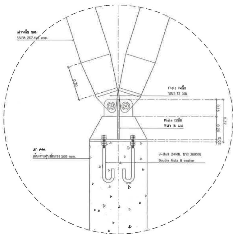
แบบขยายฐานเสารับแฉ่งระแนงตกแต่ง มาตราส่วน 1:10
