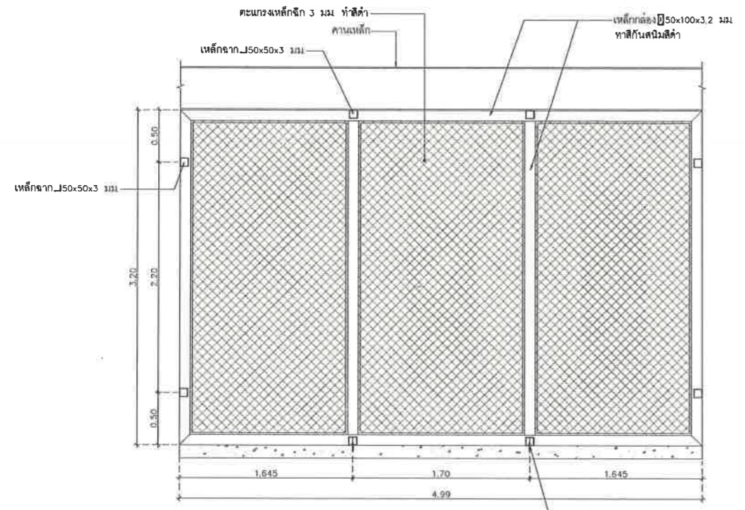
แบบขยายตะแกรงเหล็กฉีก มาตราส่วน 1:25
