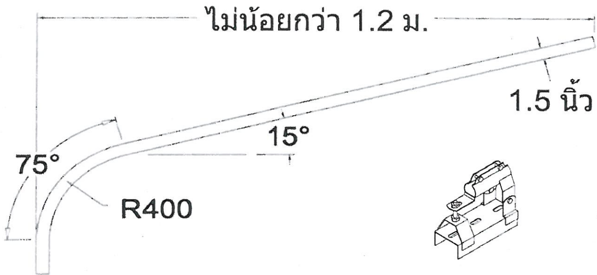
ภาพแสดงตัวอย่างรายการที่ 19 ก้านคอมไฟบอนน พร้อมขาจับ ขนาด 1.5 นิ้ว ระยะยื่น 1.20 ม.
