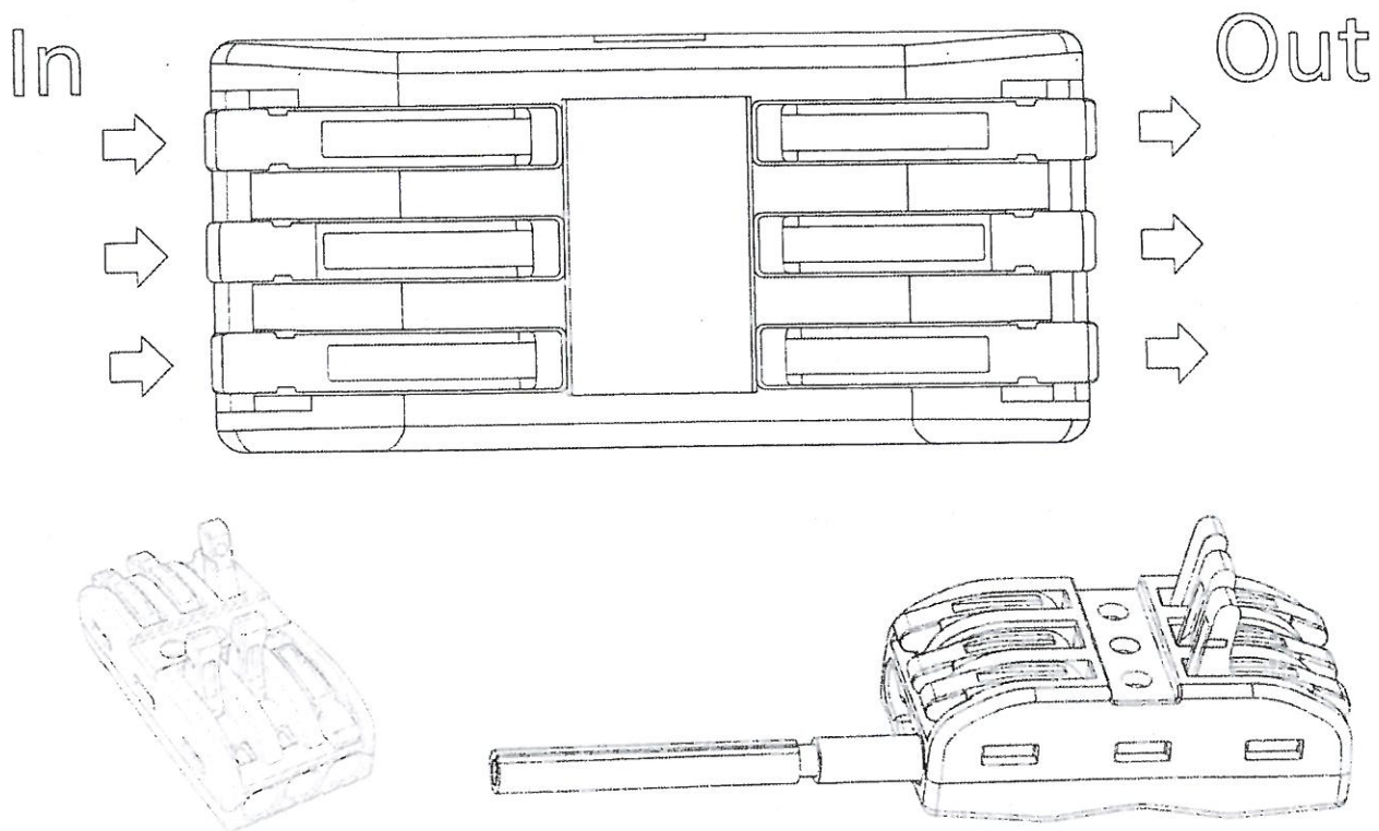
ภาพแสดงตัวอย่างรายการที่ 23 เทอร์มินอลต่อสายไฟ ชนิดก้านยก ขนาด 3-3 ช่อง
